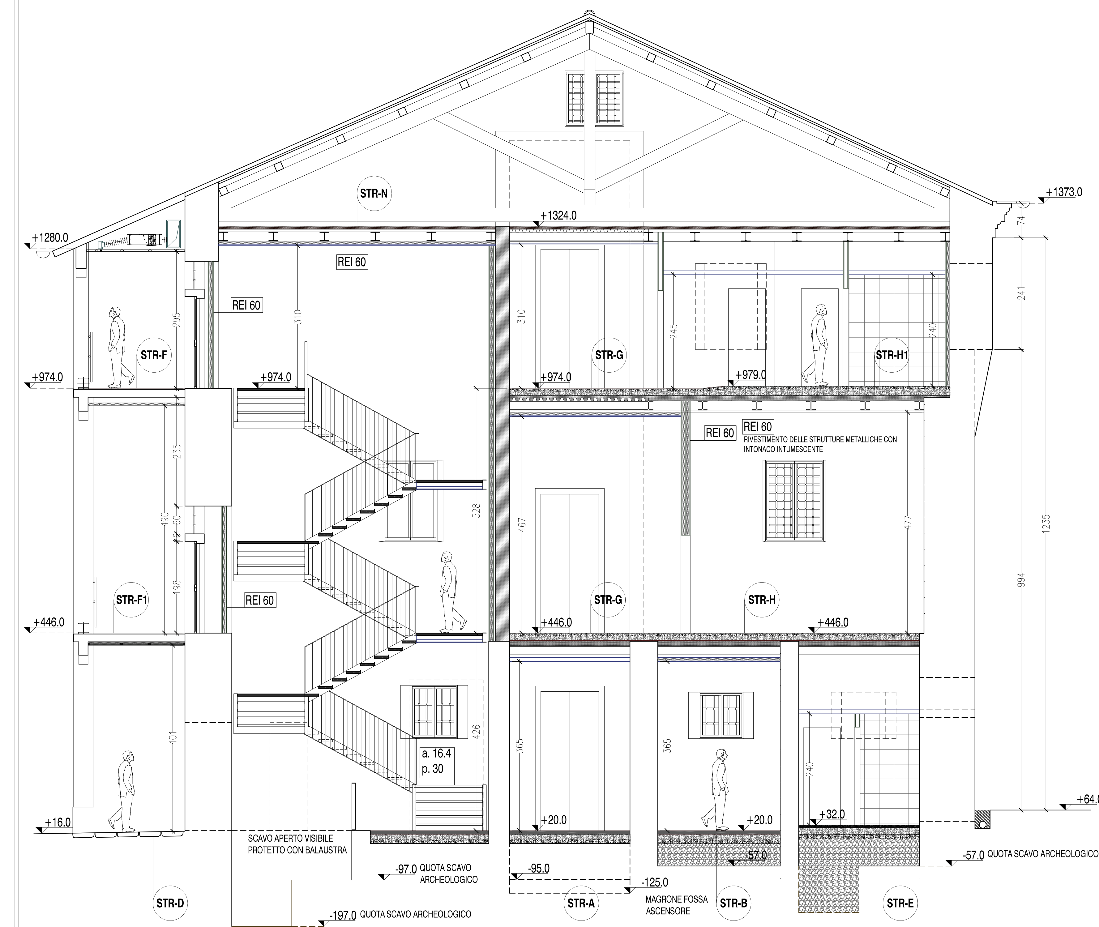
SEZIONE AA'
