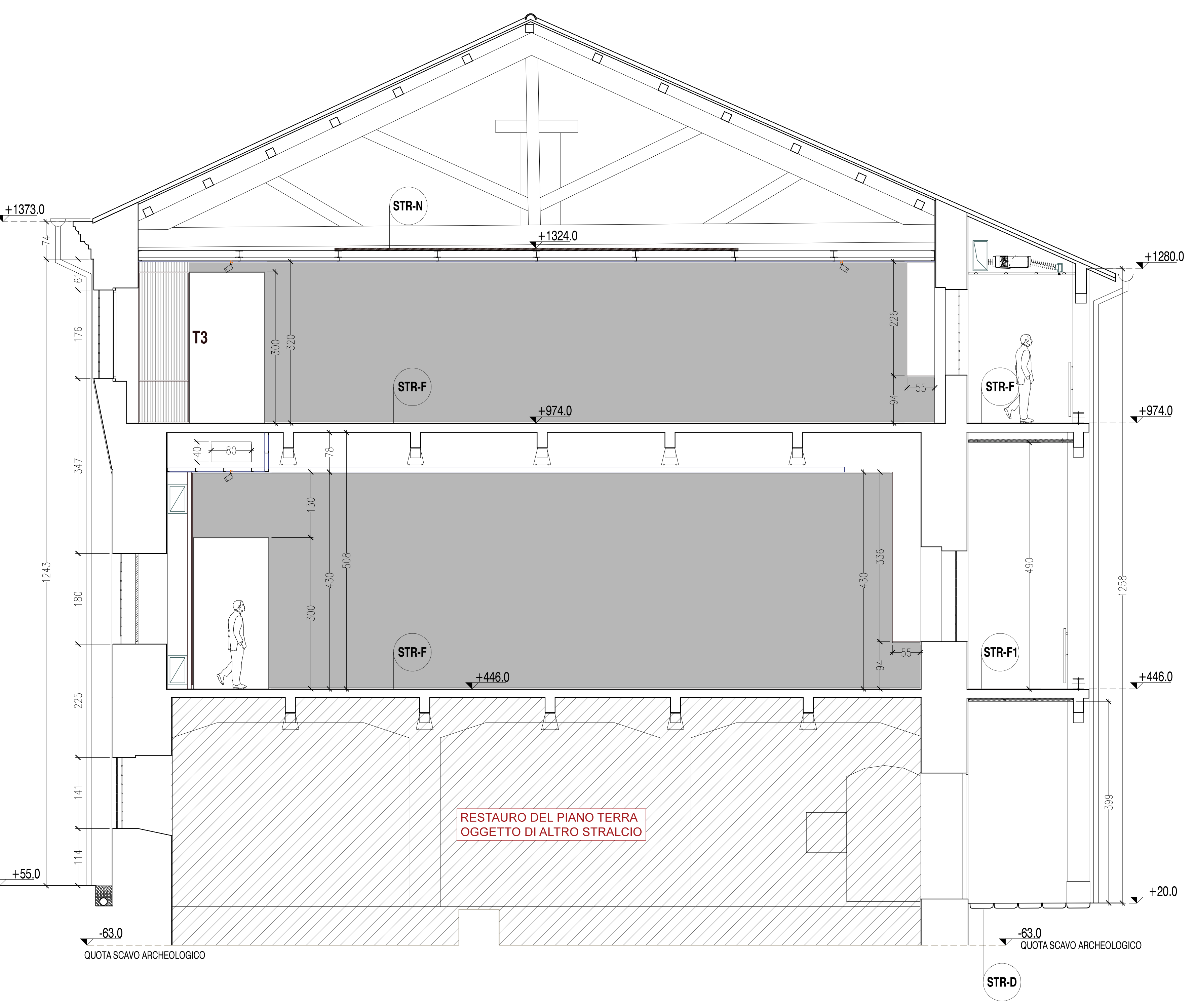
SEZIONE BB'
