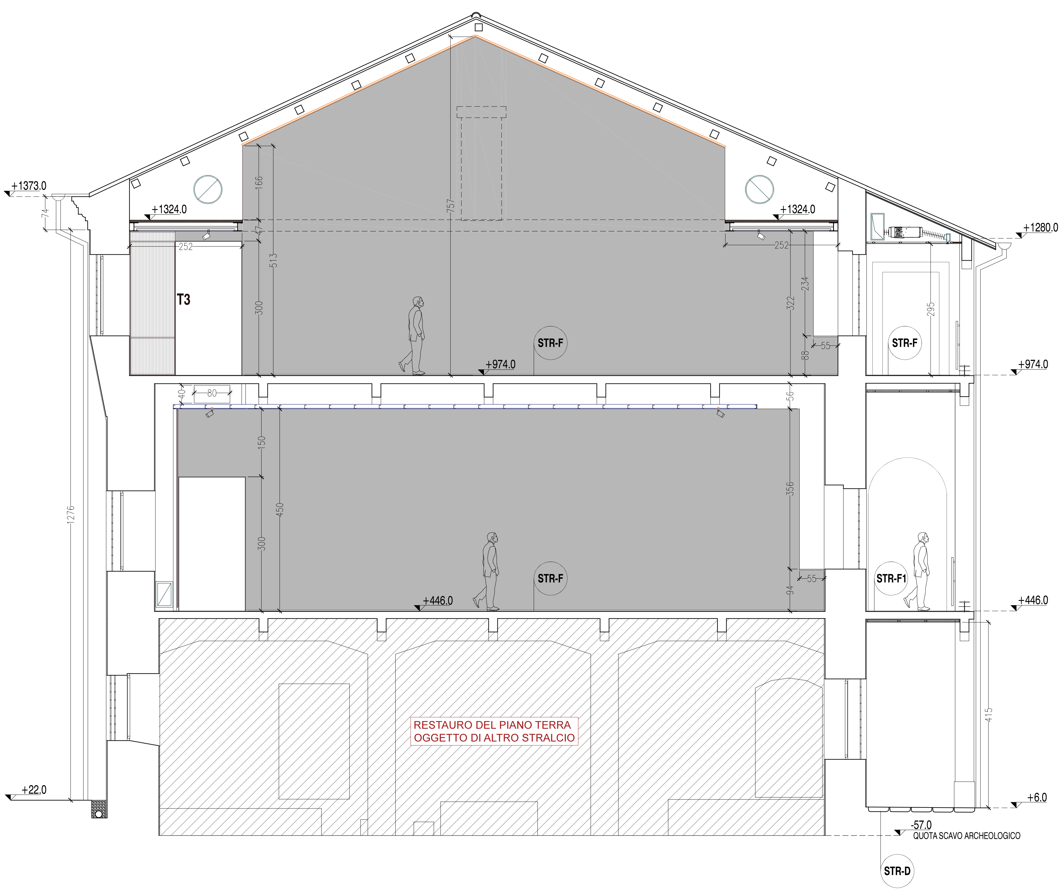
SEZIONE CC'
