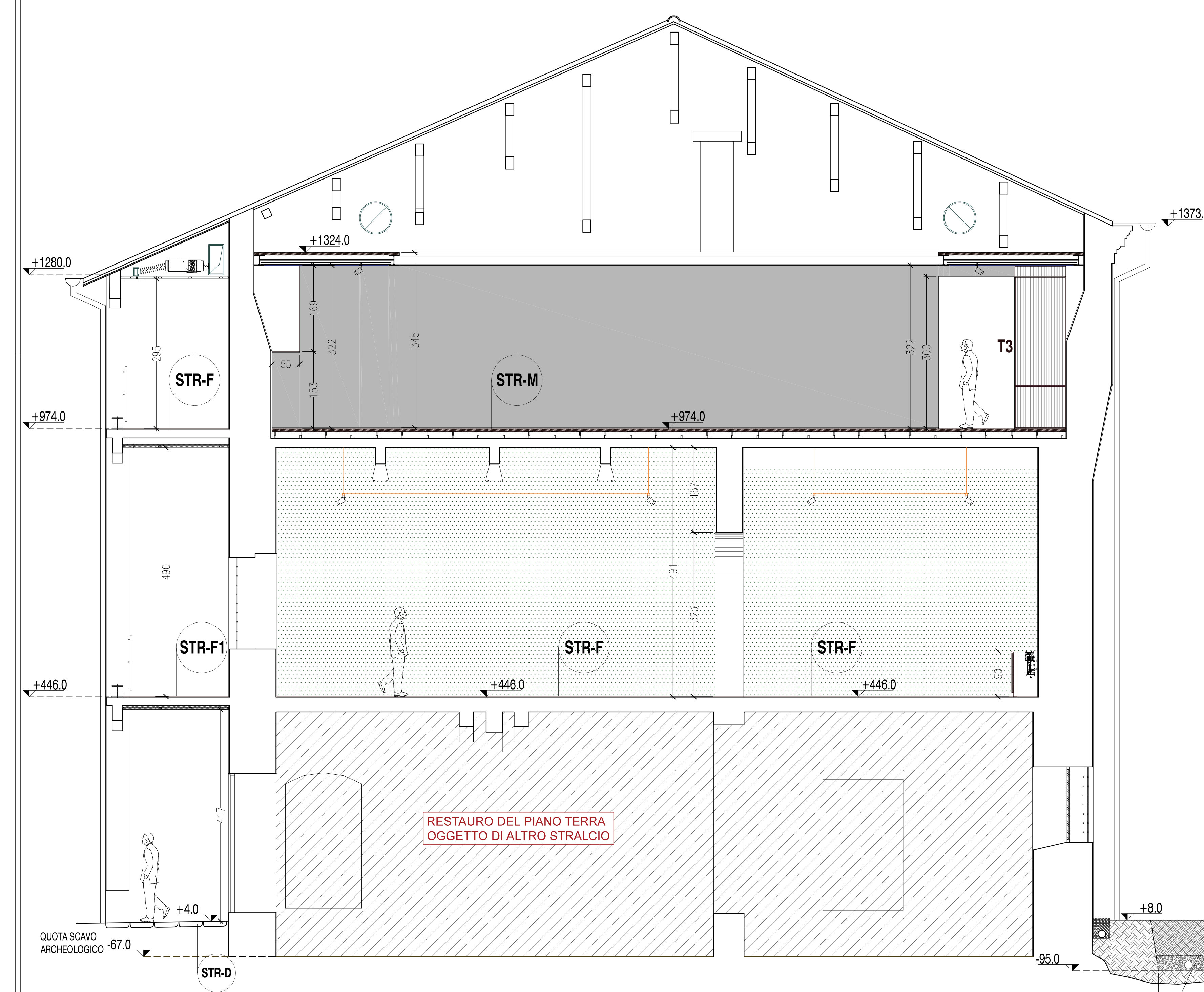
SEZIONE DD'
