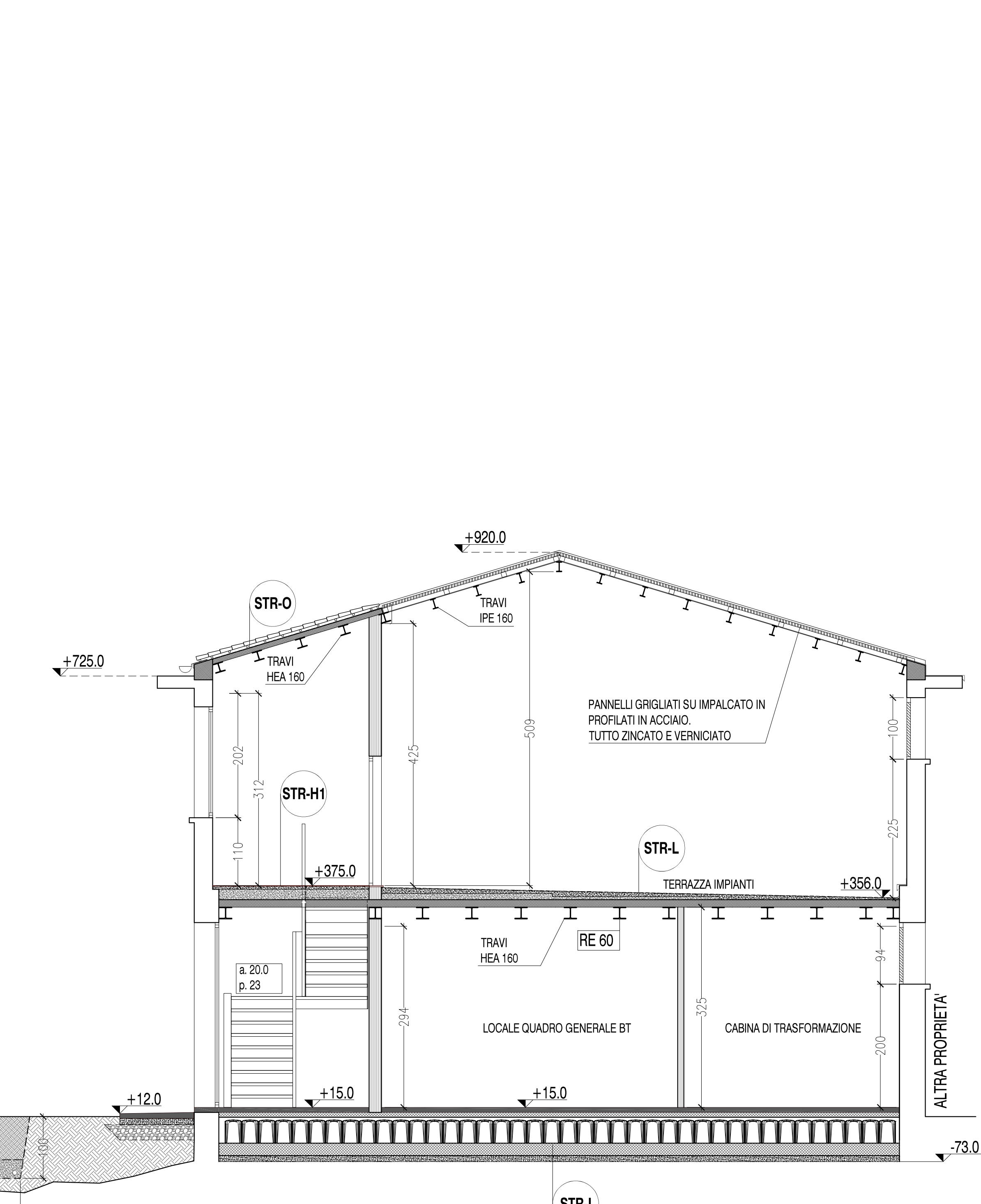
SEZIONE BB'
