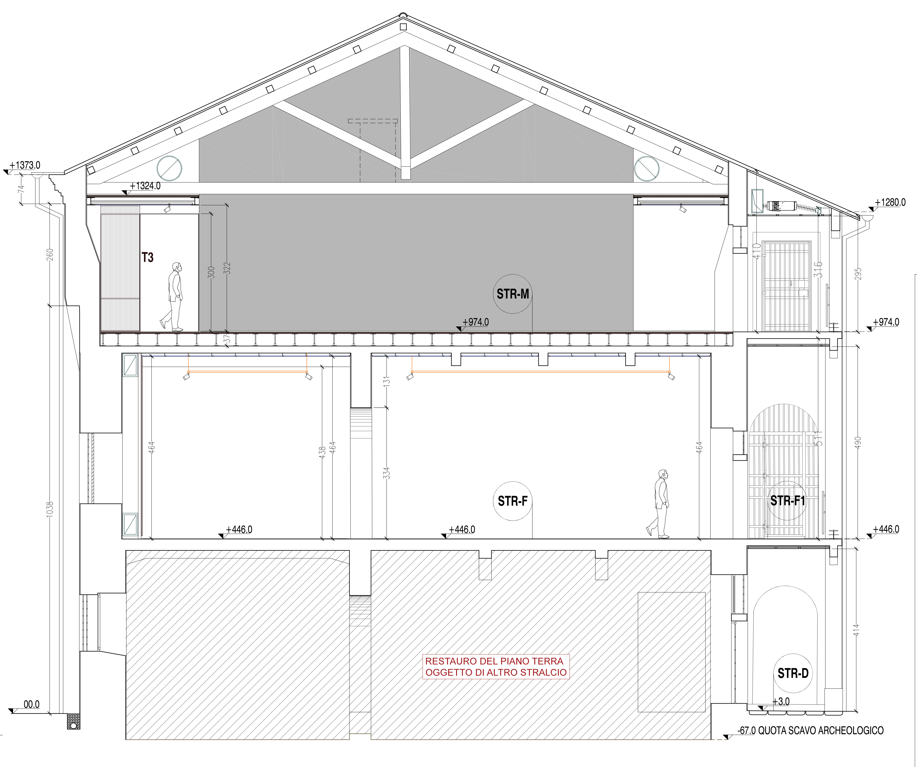
SEZIONE EE'
