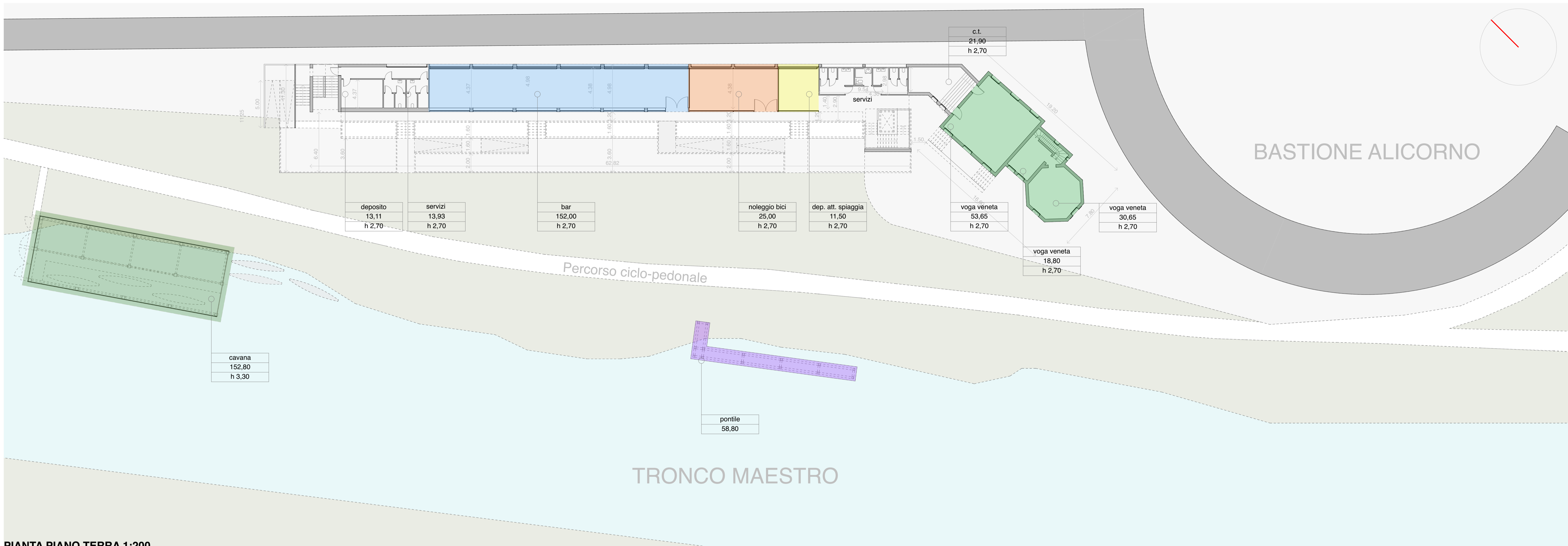
PIANTA PIANO TERRA 1:200
