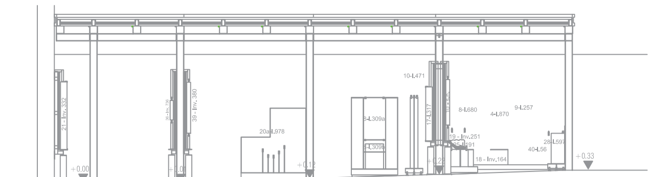
SEZIONE TRASVERSALE B-B - PIANO TERRA - Scala 1:100
