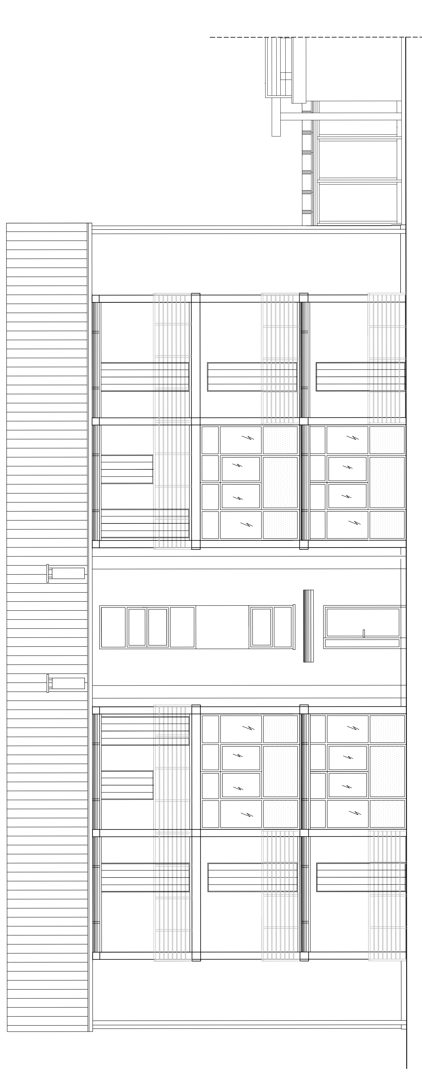
PROSPETTO OVEST
