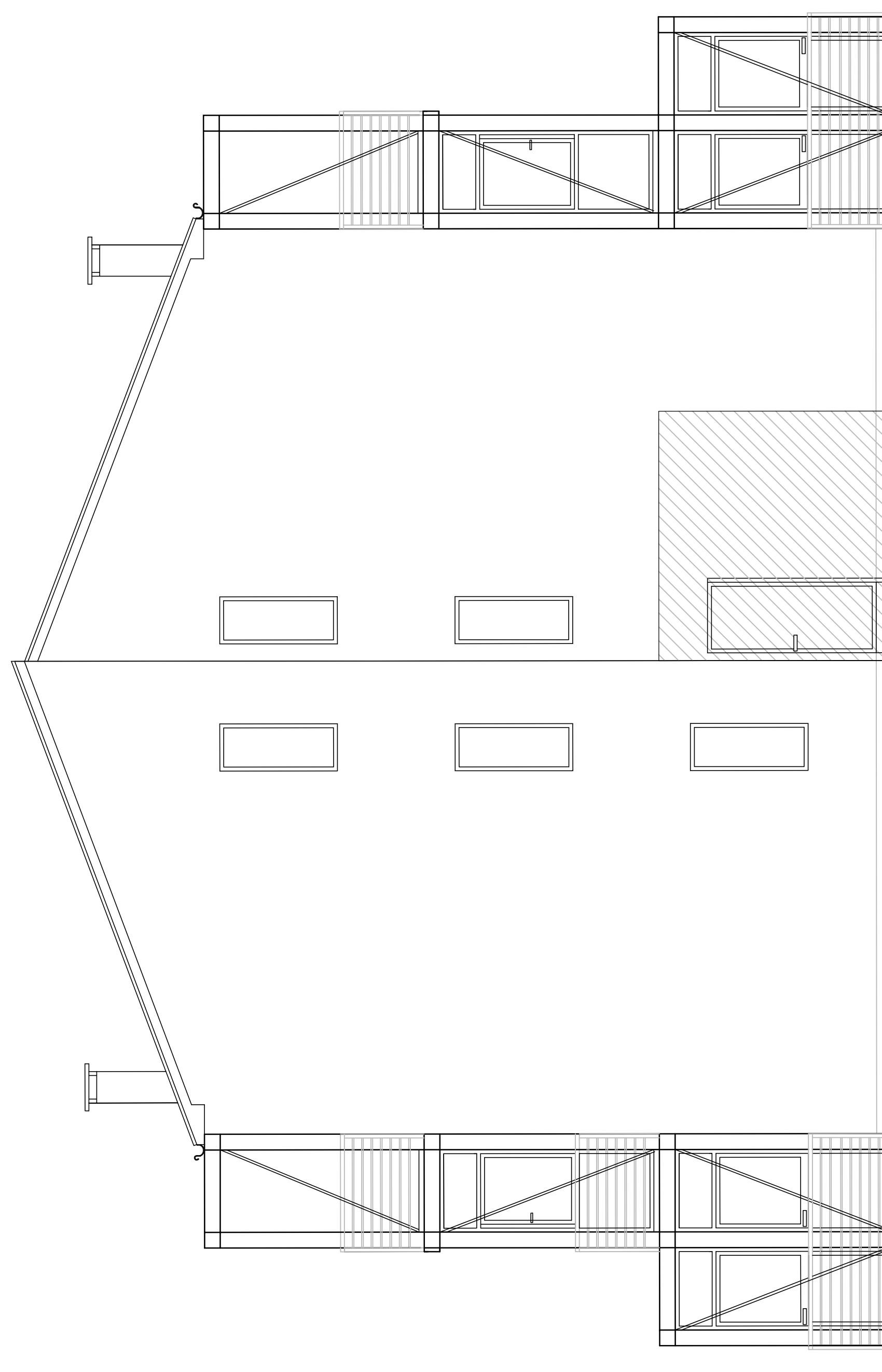
PROSPETTO SUD
