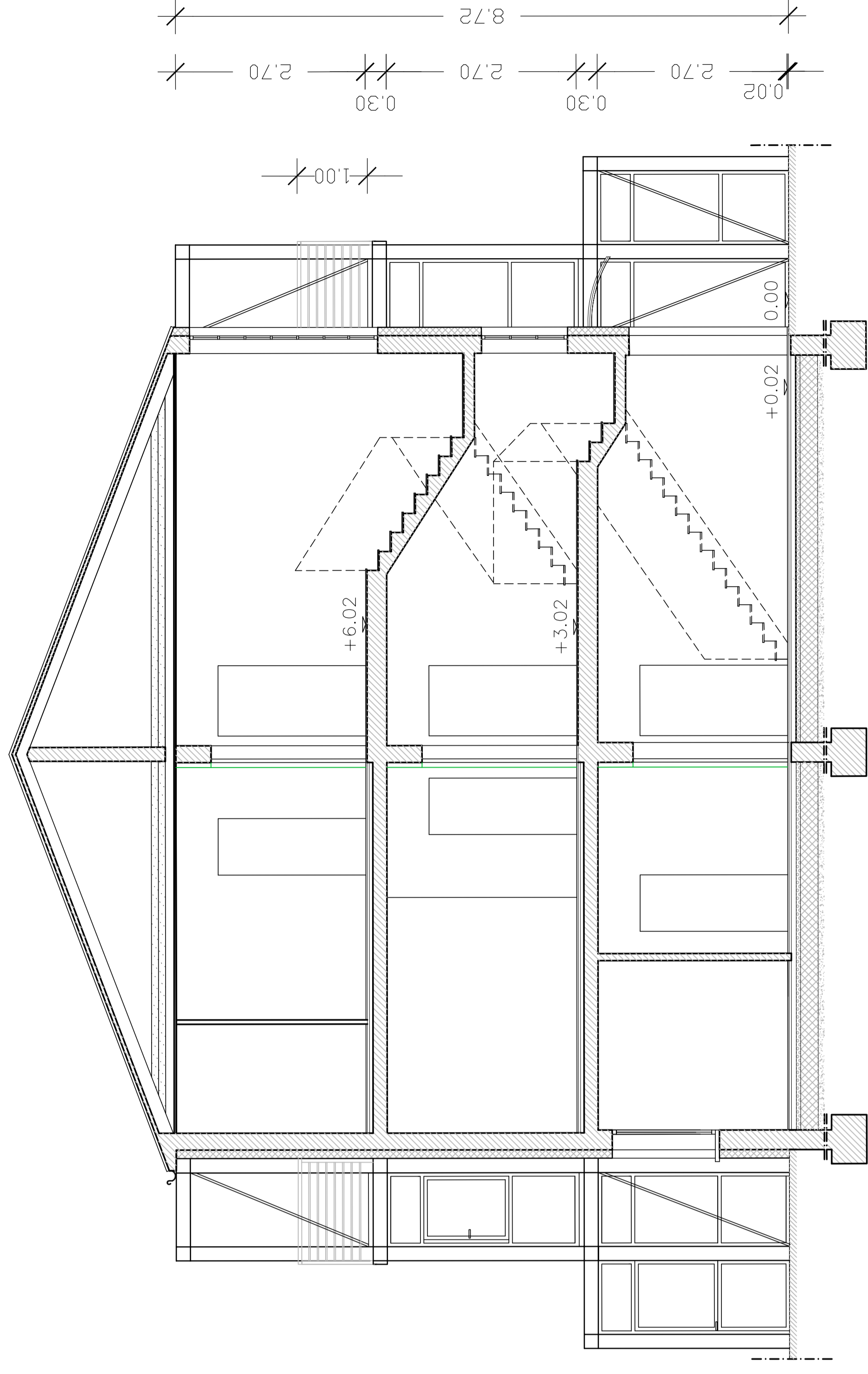
SEZIONE C-C
