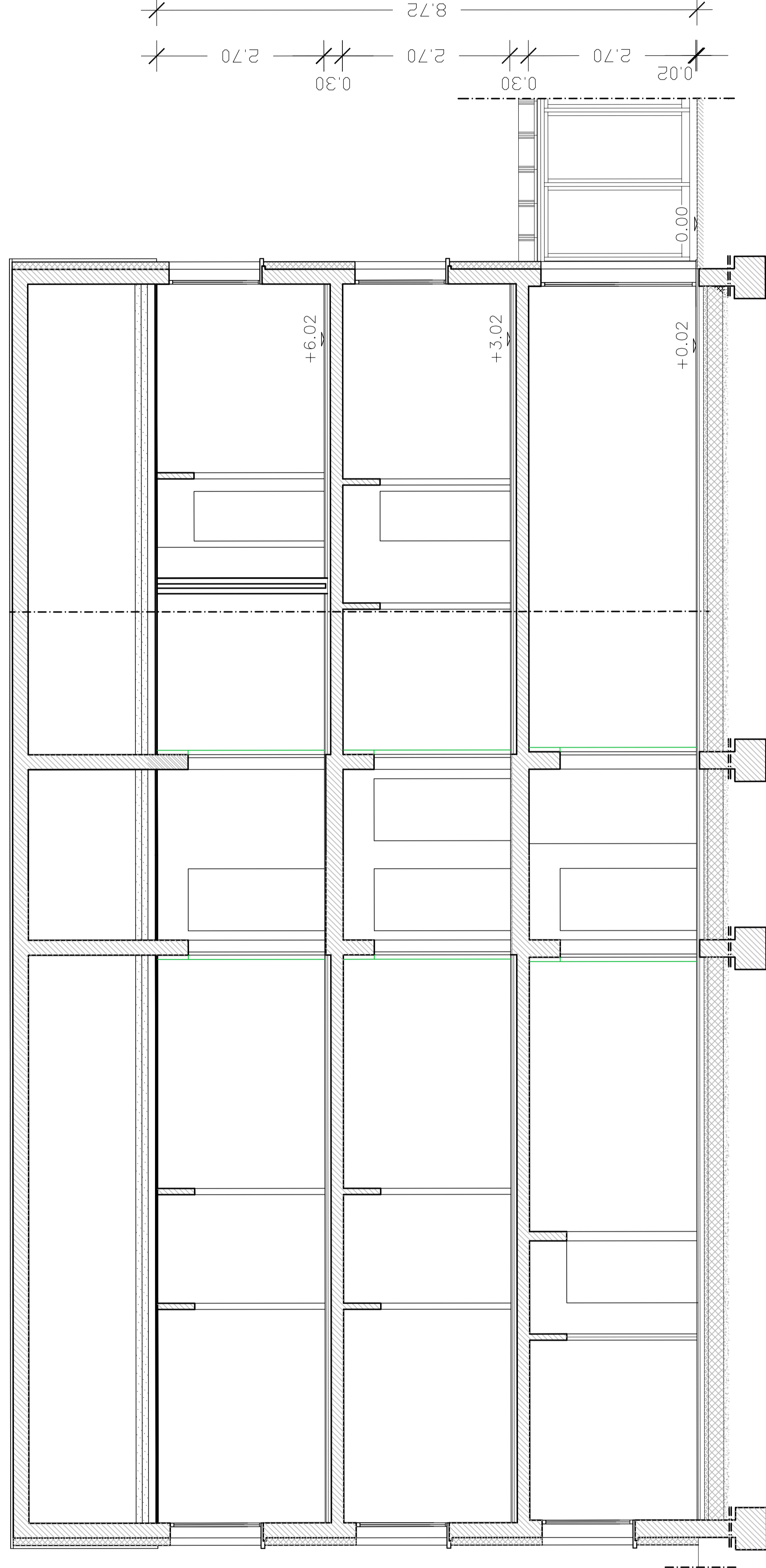
SEZIONE B-B
