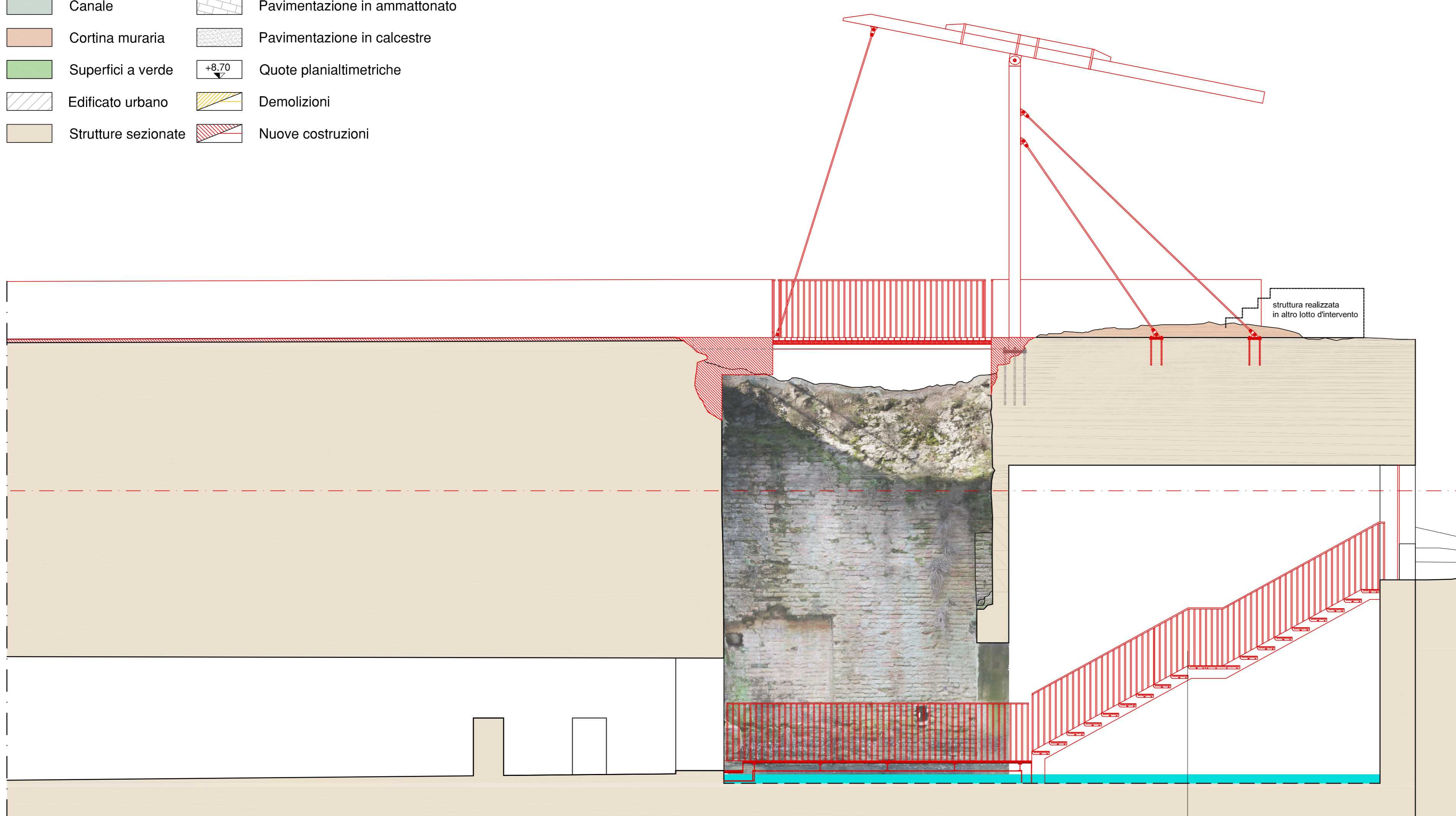
SEZIONE A-A'
