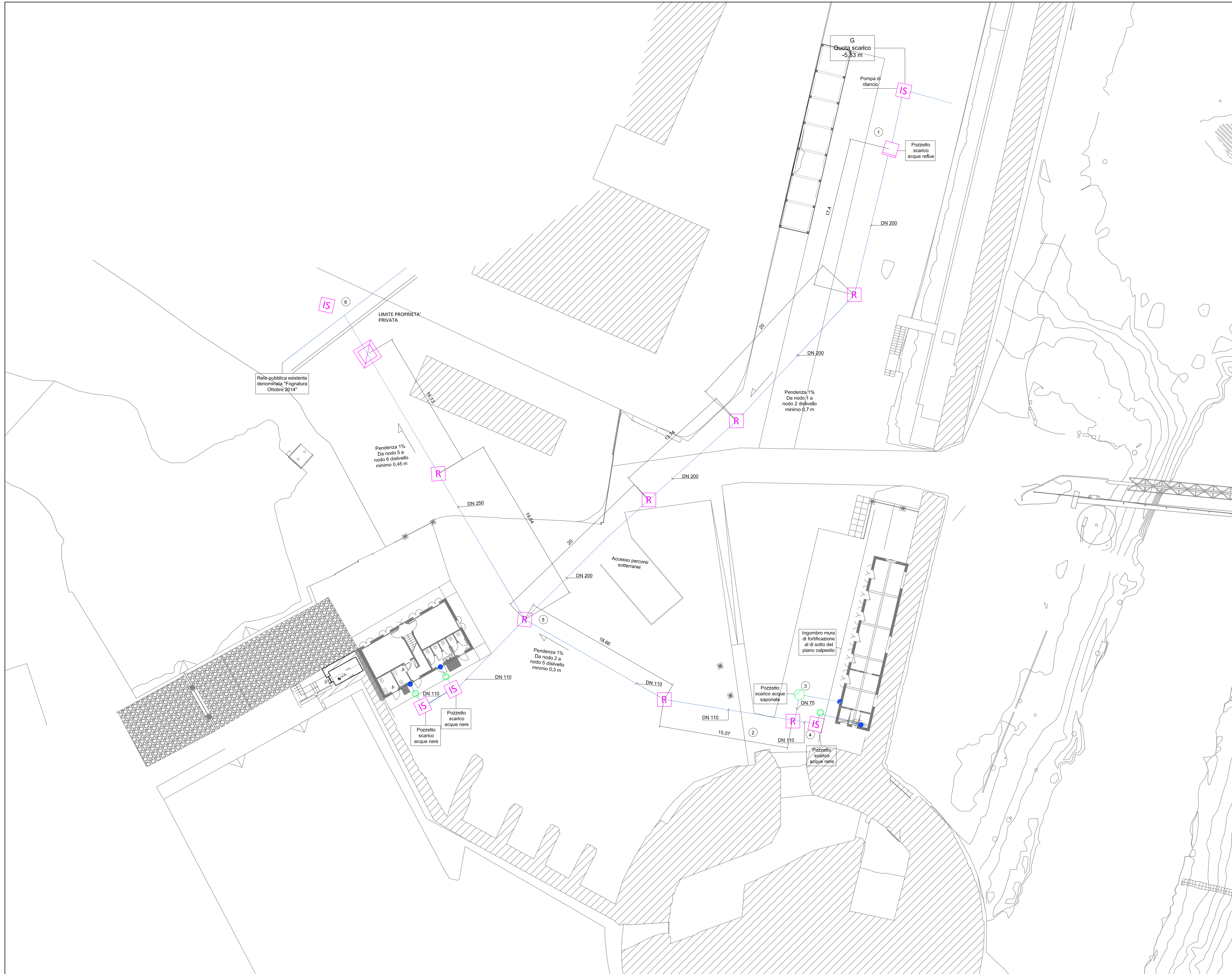
Planimetria Impianto di convogliamento scarichi alla rete pubblica e scarichi condensa
