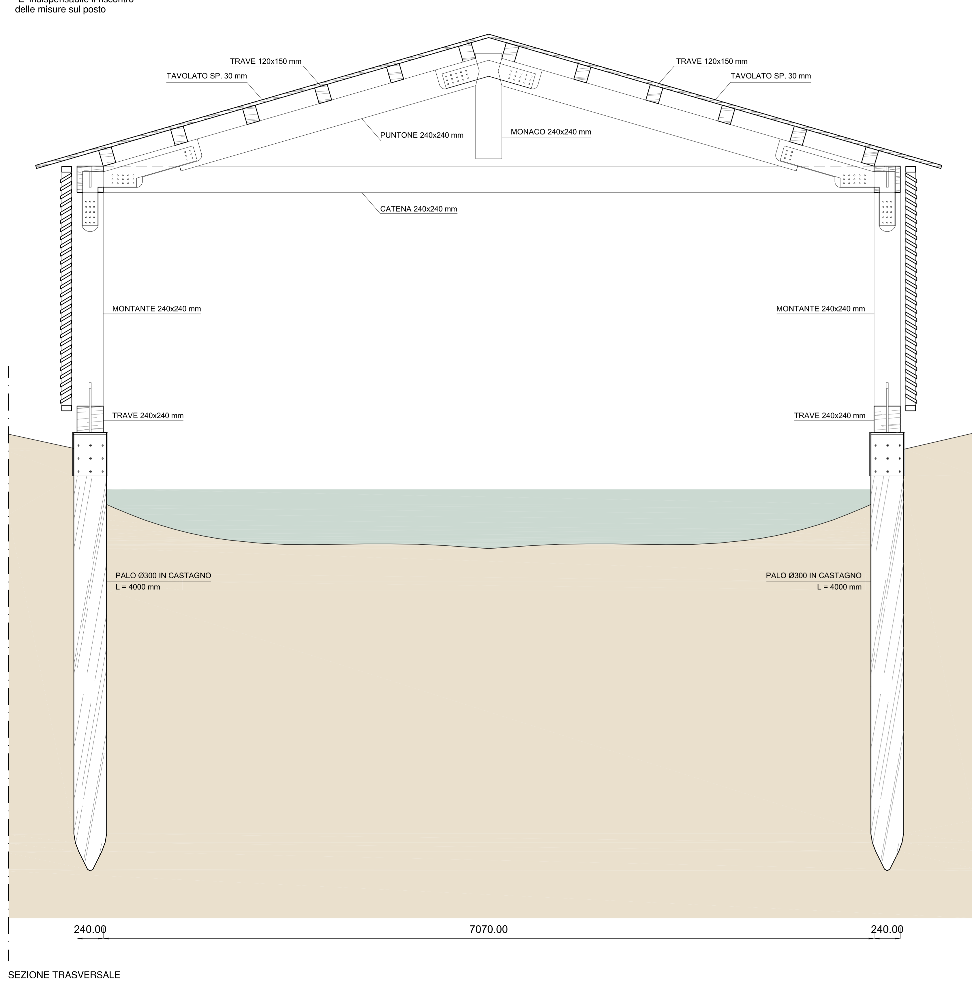
SEZIONE TRASVERSALE
