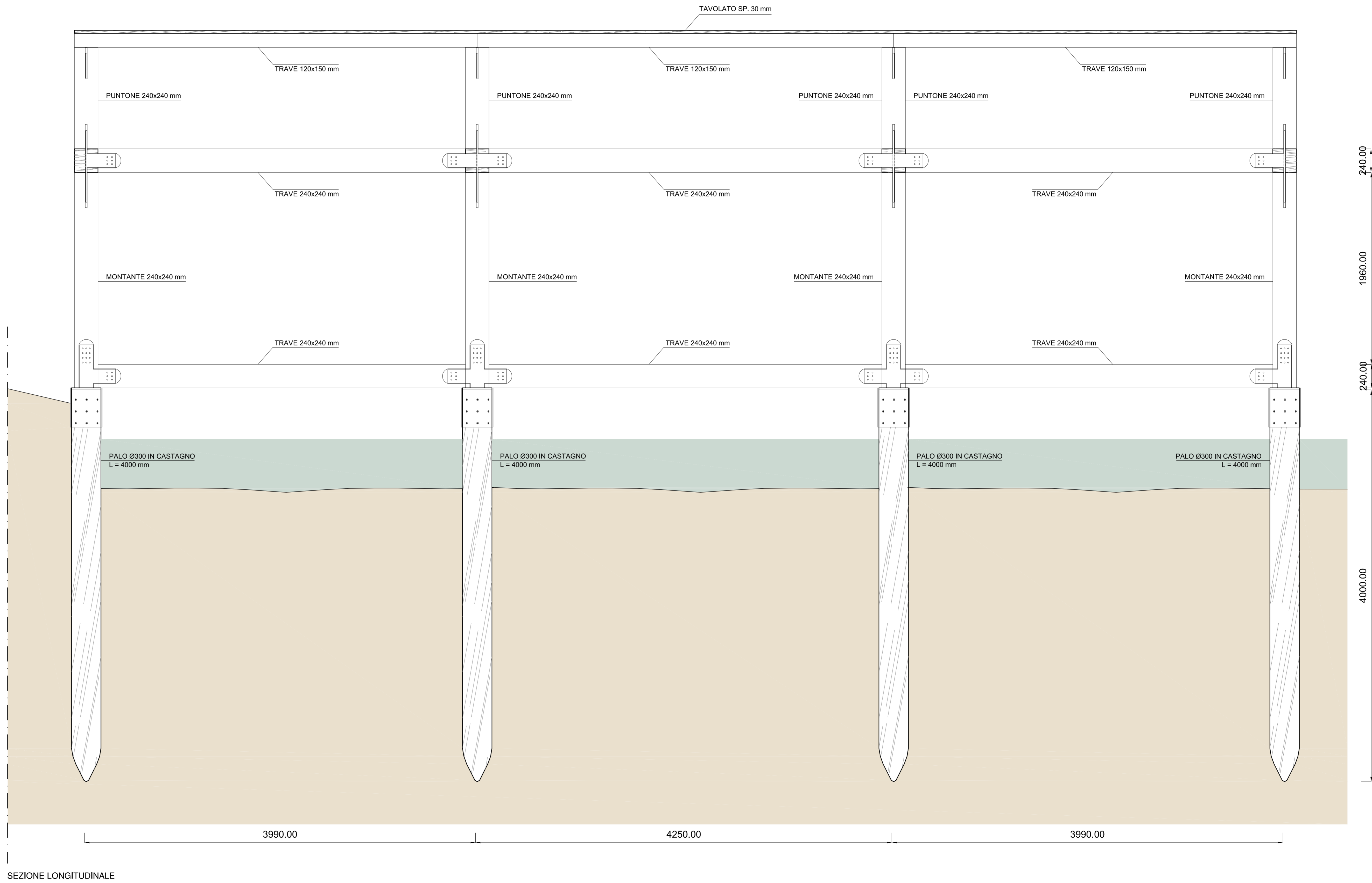
SEZIONE LONGITUDINALE
