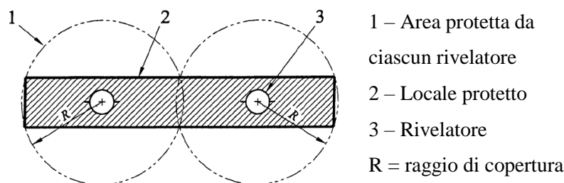
Figura 4 - Corretta installazione di rivelatori in locali aventi lati tra loro diversi.
