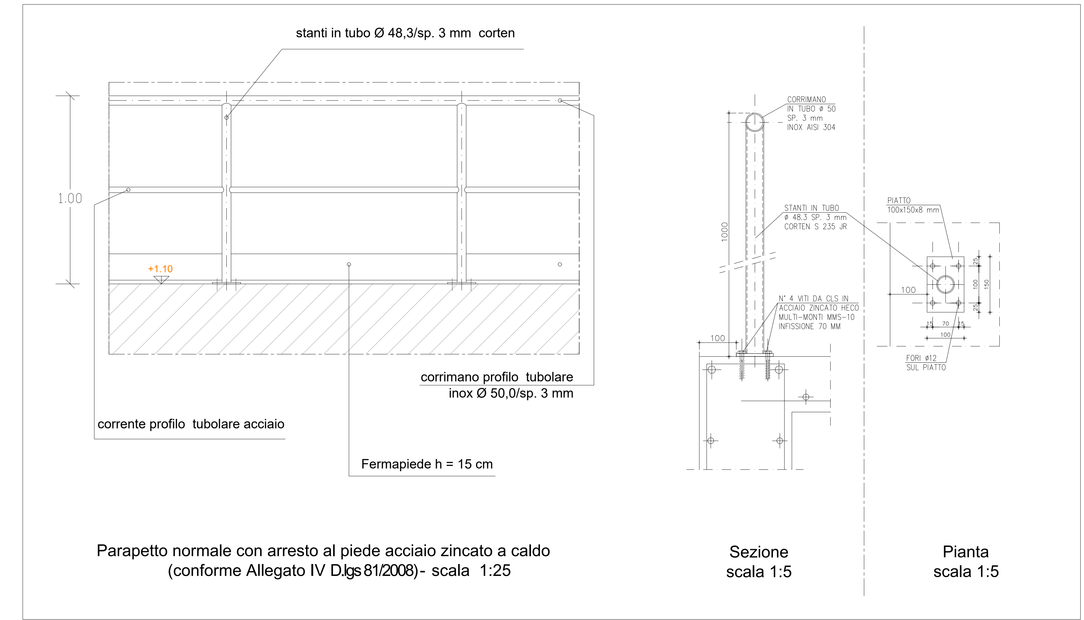
Parapetto banchine tipo - scala 1:25 / scala 1:5
