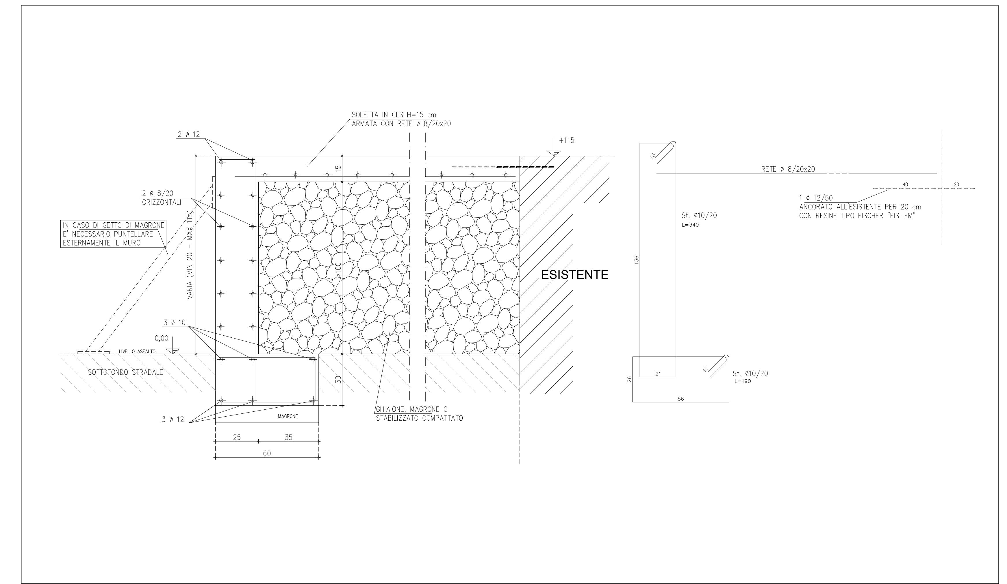
Particolare muro di contenimento e soletta per nuova rampa - scala 1:25
