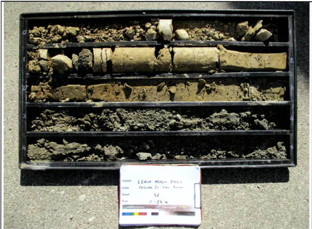
Sondaggio S2 – Cassetta N. 1 : da 0.0 m a 5.0 m
