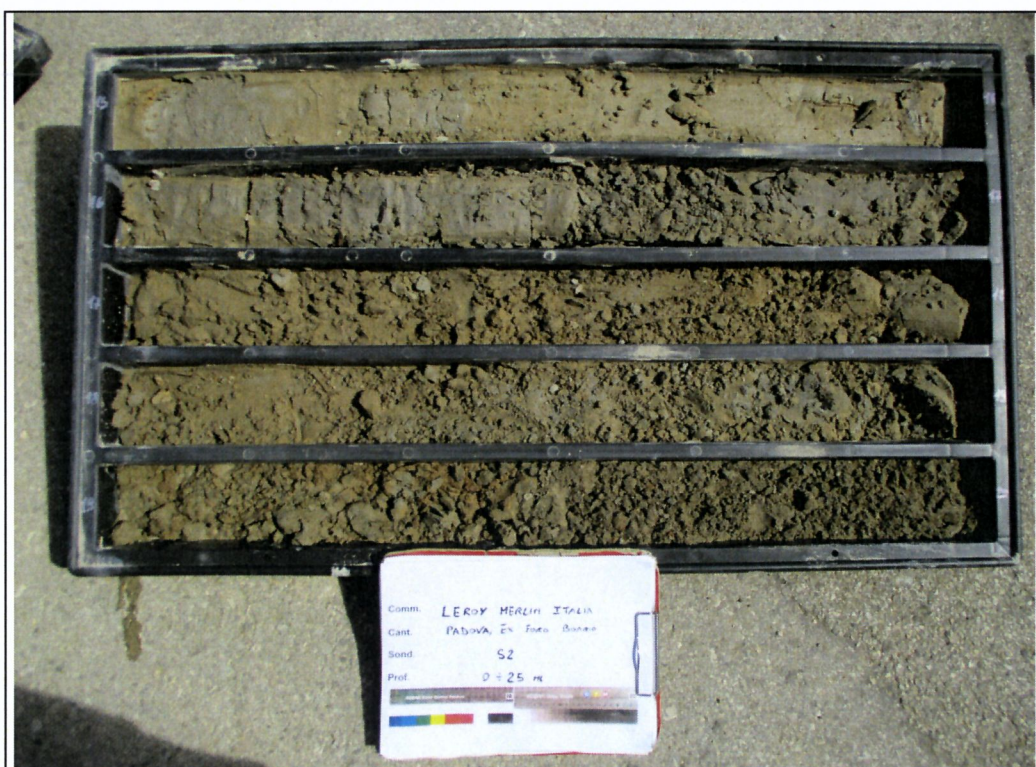
Sondaggio S2 – Cassetta N. 4 : da 15.0 m a 20.0 m
