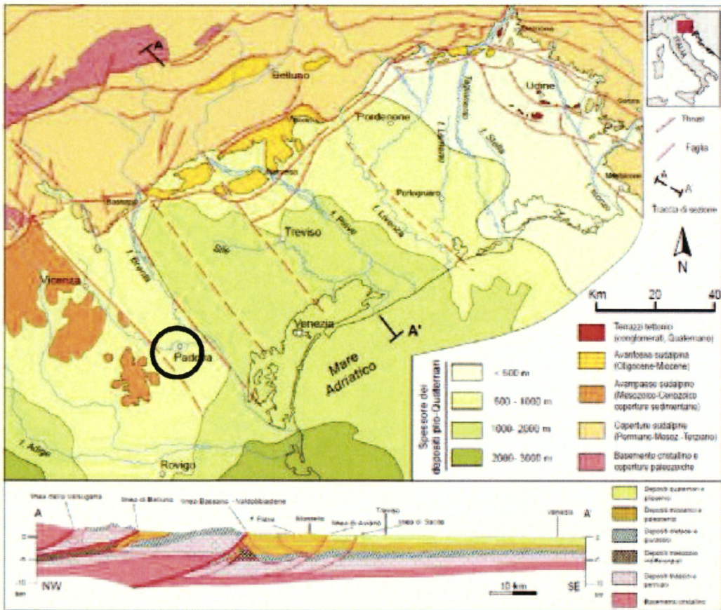
SCHEMA GEOLOGICO-STRUTTURALE DELLA PIANURA VENETA
