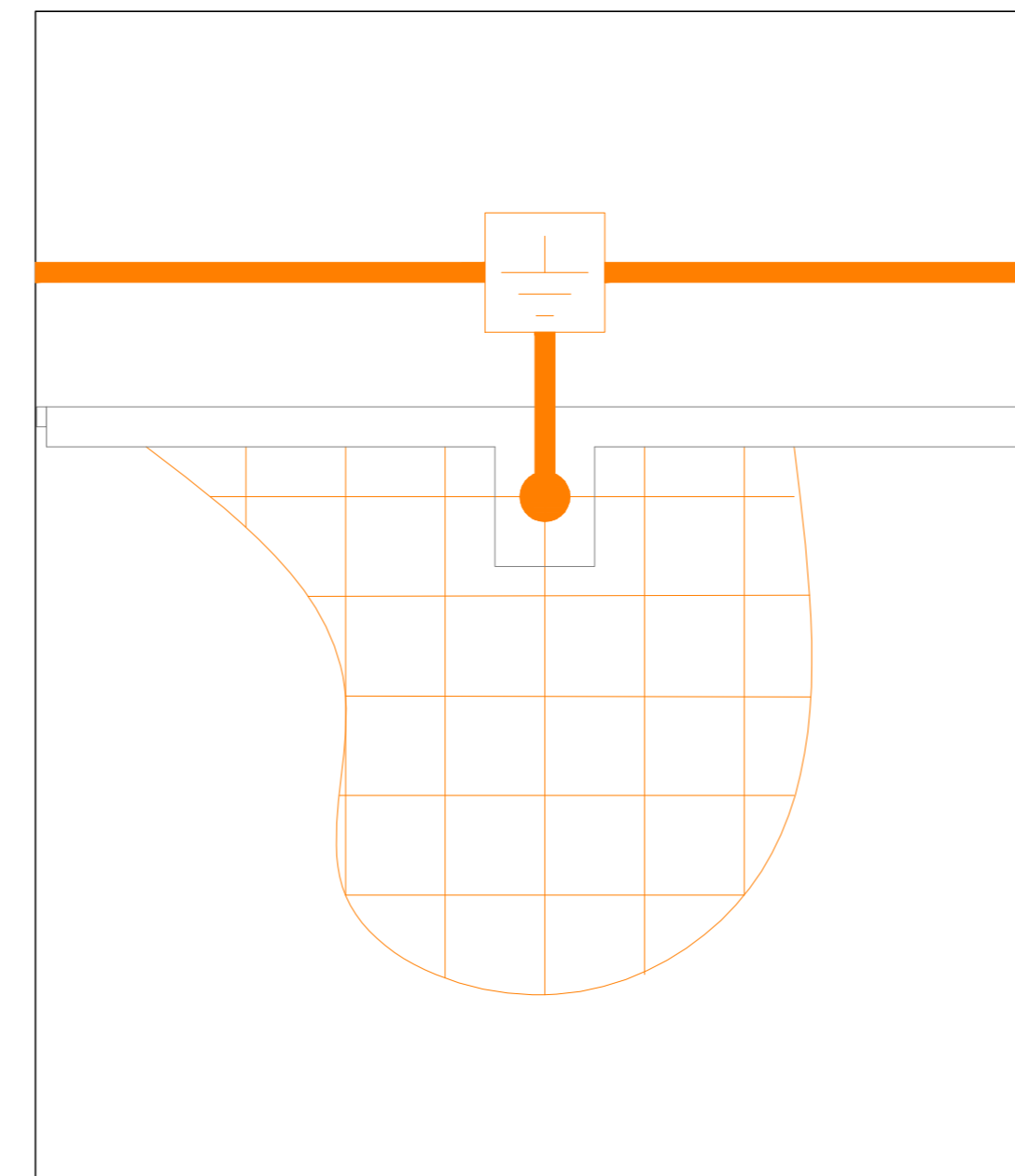
PARTICOLARE COLLEGAMENTO A TERRA RETE ARMATURA Scala 1:100
