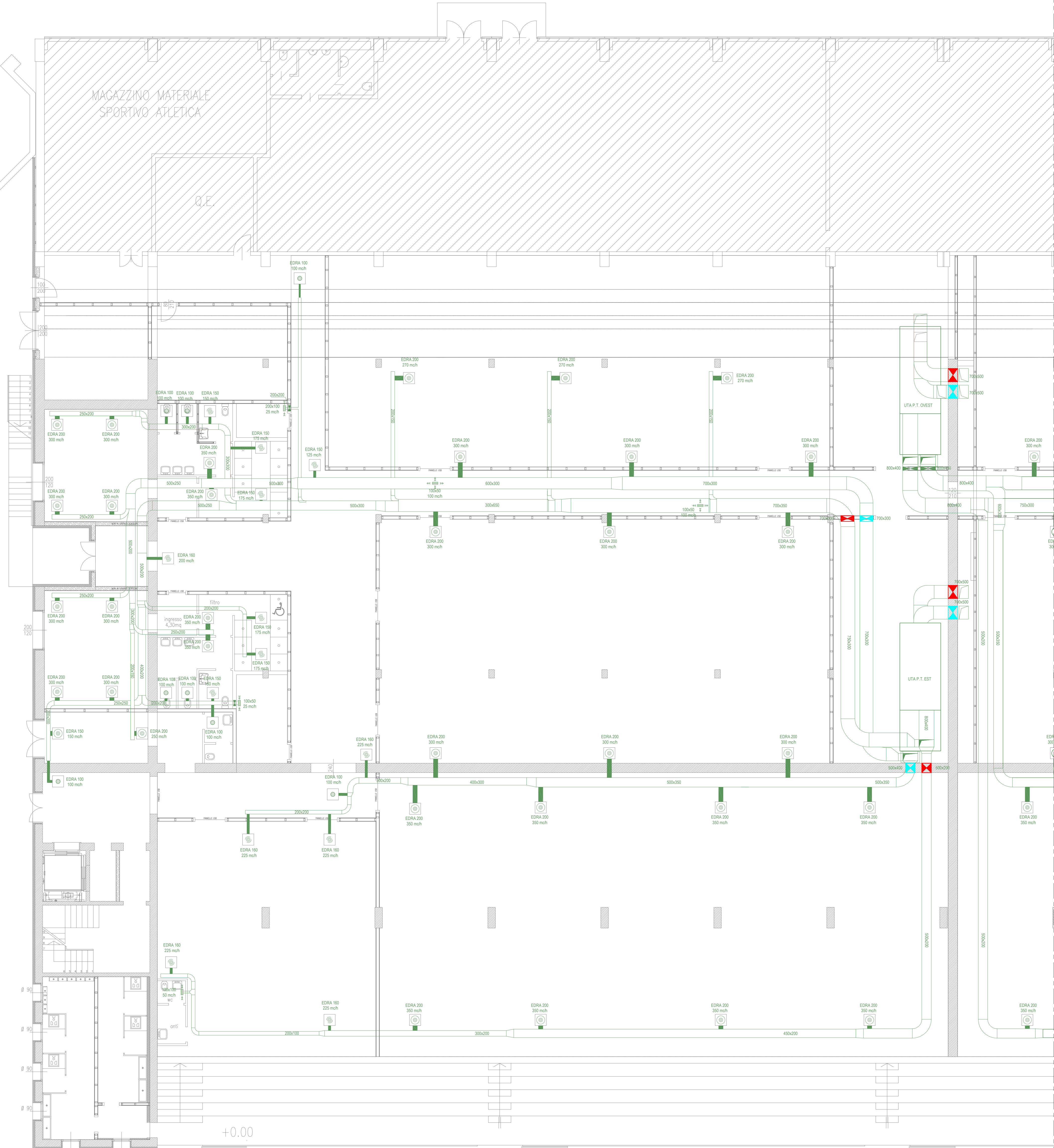
DISTRIBUZIONE ARIA PIANTA EST QUOTA +0,00 SCALA 1:100
