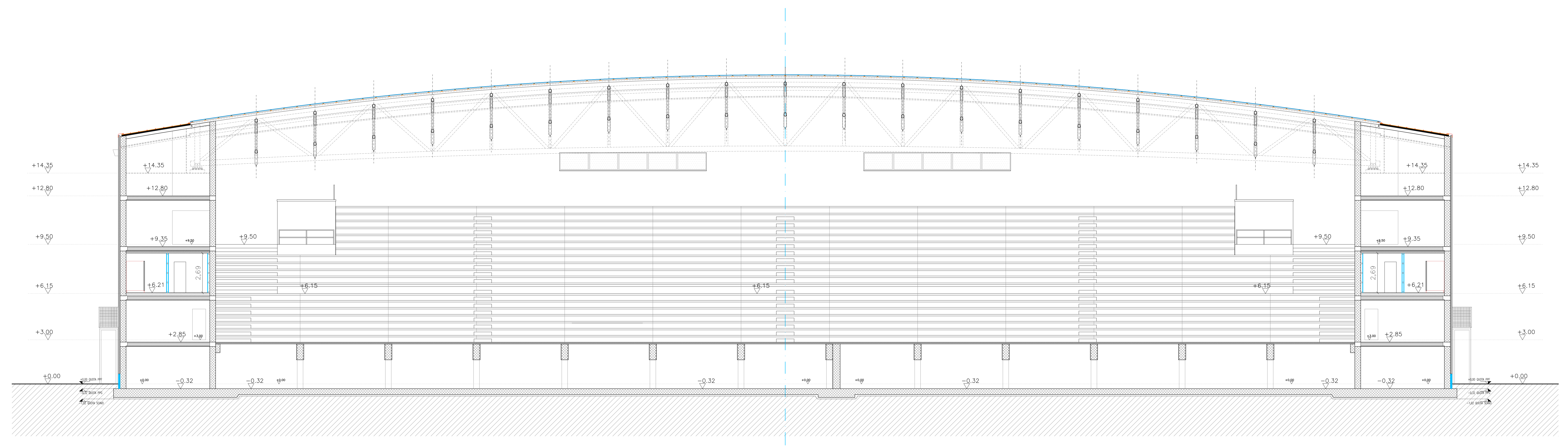
SEZIONE C-C
