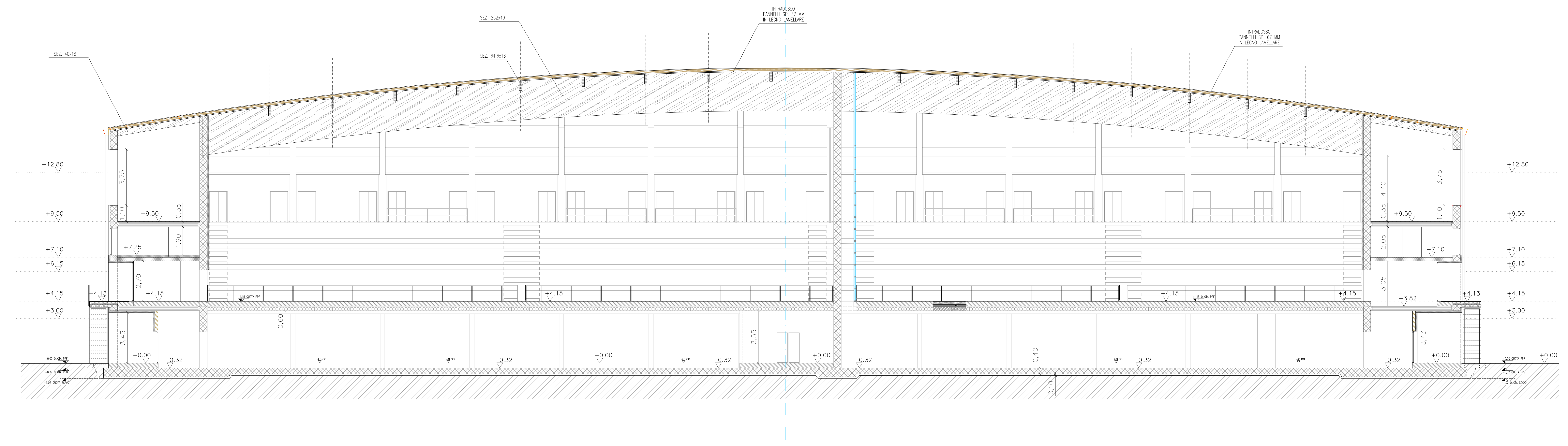
SEZIONE D-D
