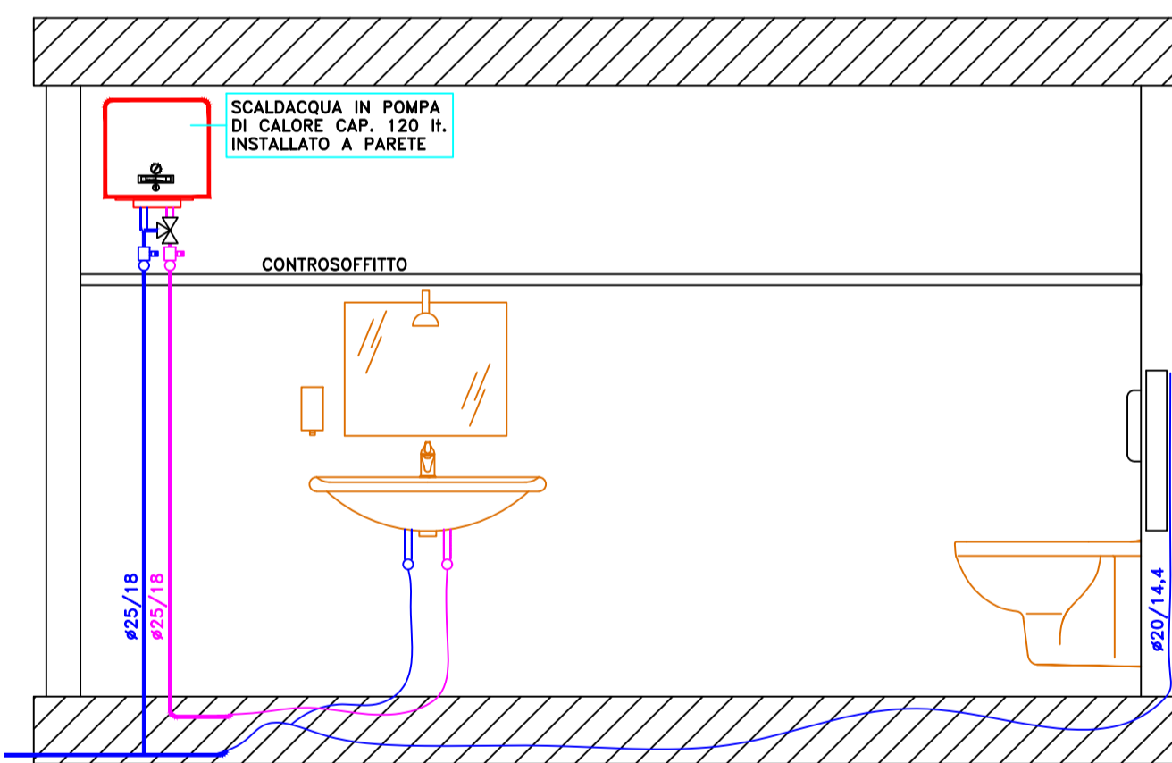
SCHEMA VERTICALE
