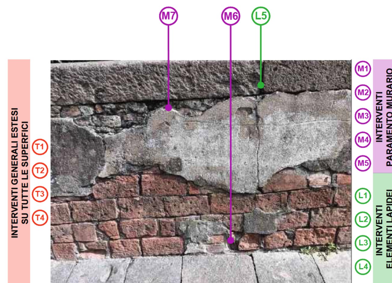
PARAPETTO INTERNO A VALLE
