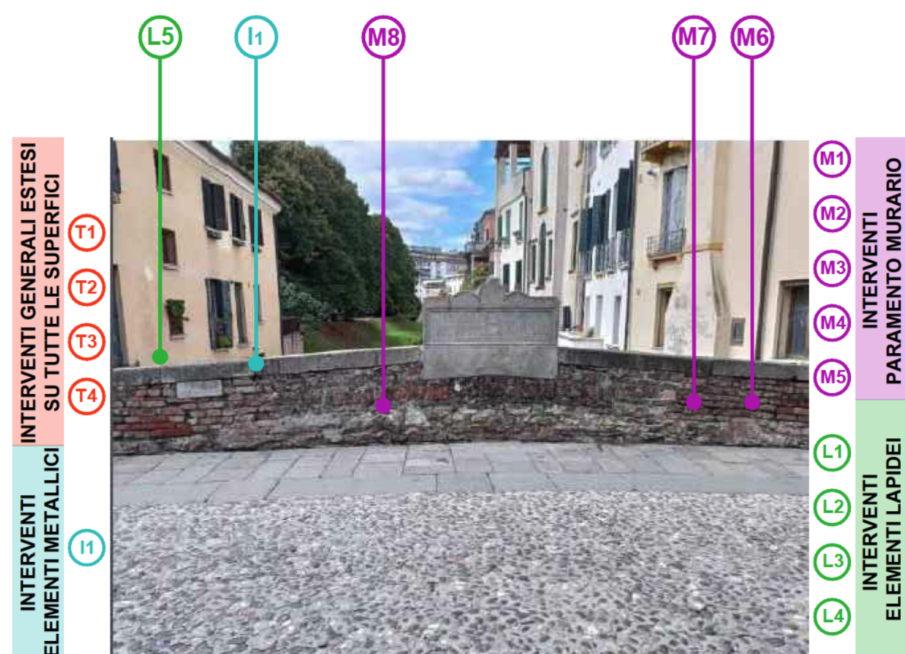
PARAPETTO INTERNO A MONTE
