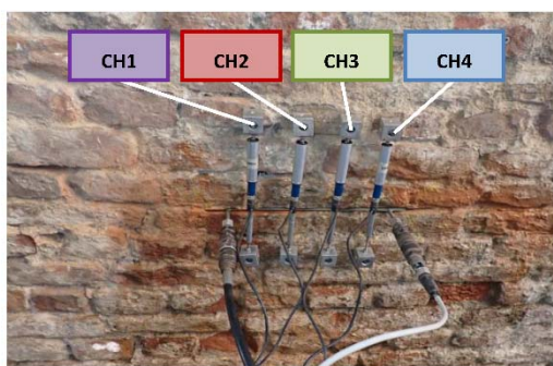
Schema dei sensori durante la prova
