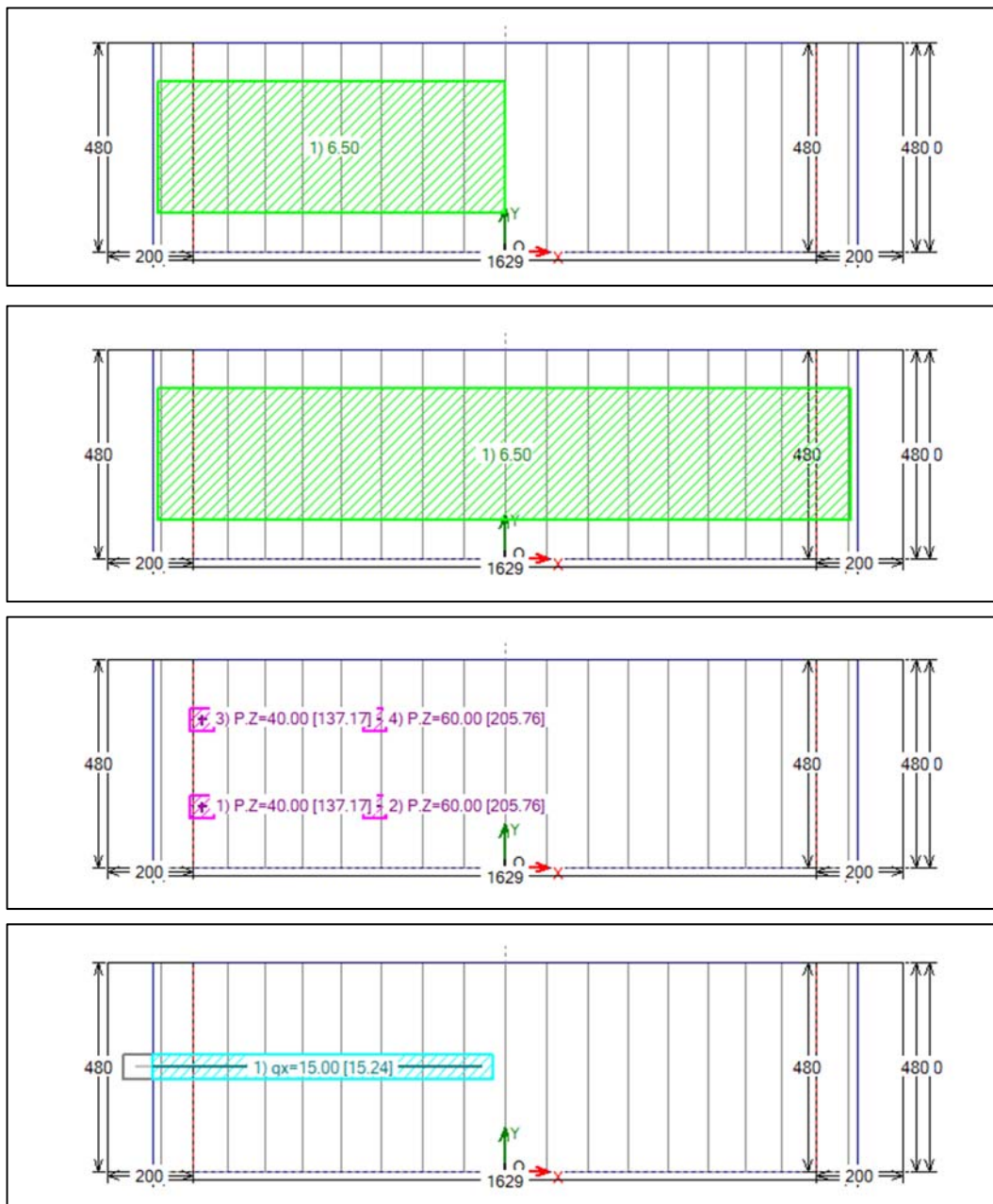
Fig. 28 Vista in pianta con carichi da veicoli in transito 20t – diffusi con estensione parziali/totale e concentrati verticali e da frenamento da mezzo di progetto (kN/m).
