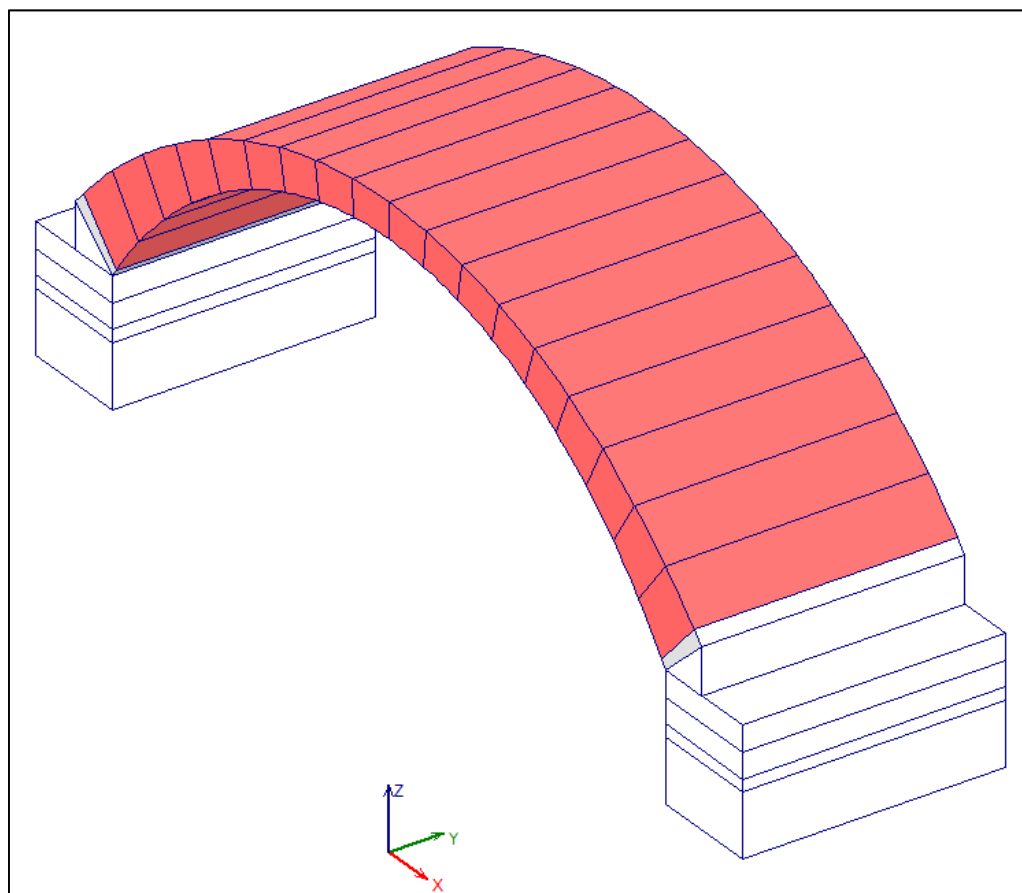
Fig. 22 Rappresentazione 3D del modello a conci.
