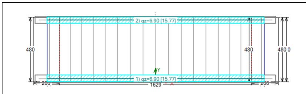
Fig. 26 Vista in pianta con carichi lineari dovuti ai muri di coronamento (kN/m).
