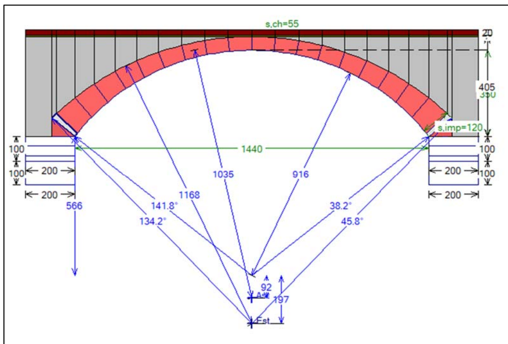
Fig. 23 Geometria degli elementi portanti in muratura (cm) con rinfianchi e rappresentazione schematica del sottofondo e della pavimentazione.
