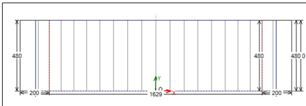
Fig. 24 Vista del modello dall'alto del manufatto (cm).
