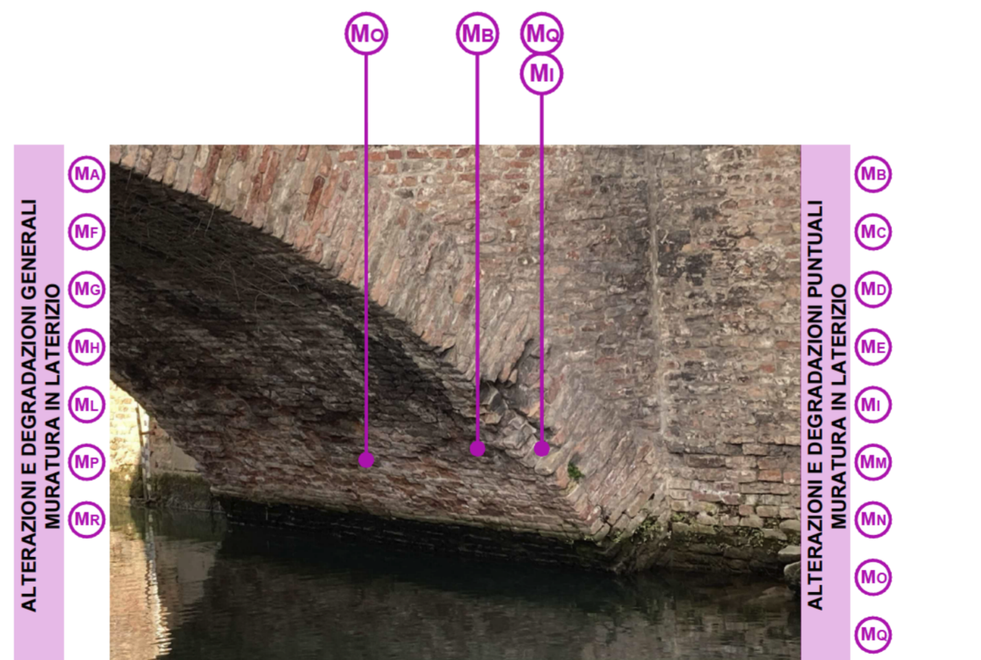
PARTICOLARE SPALLA DI VALLE IN SINISTRA
