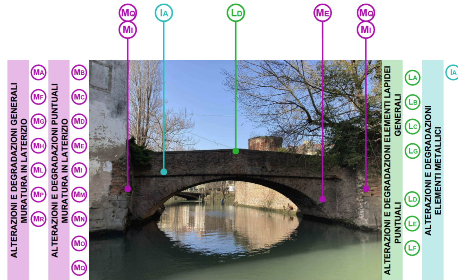
PROSPETTO DI VALLE
