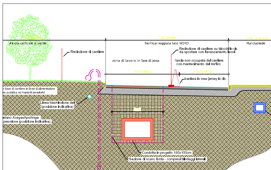
Esempio di recinzione di cantiere
