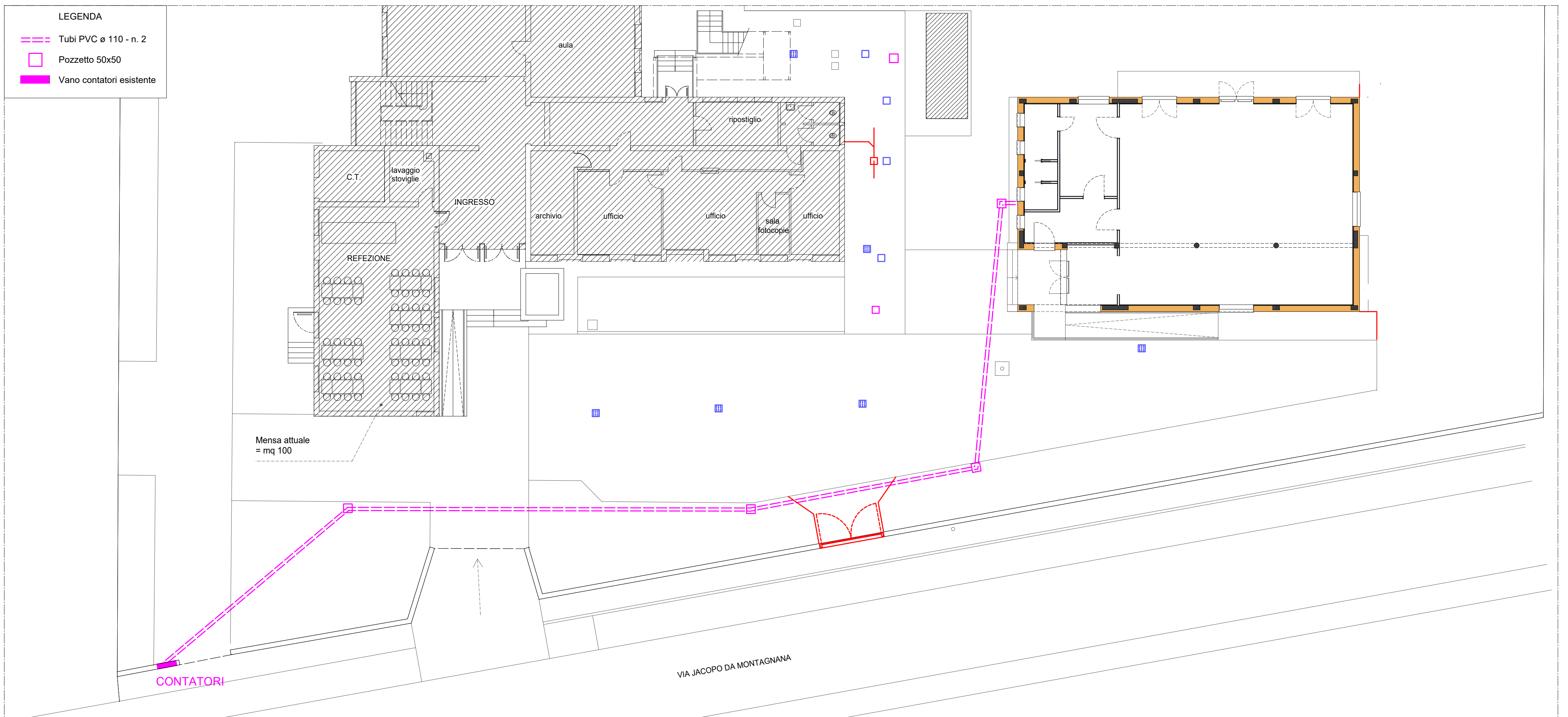
ALLACCIO RETE ELETTRICA (ENERGIA E FOTOVOLTAICO)_SCALA 1:150
