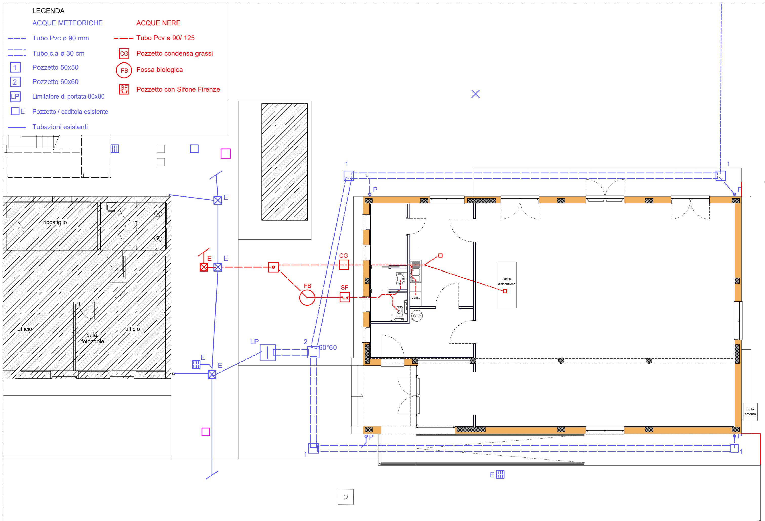
RETE FOGNATURA ACQUE METEORICHE E ACQUE NERE_SCALA 1:100
