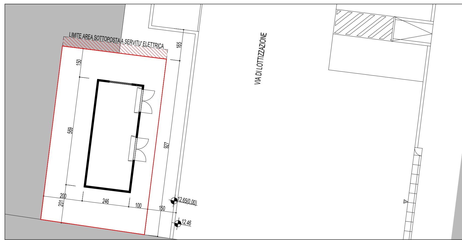
STRALCIO PLANIMETRIA CON INSERIMENTO DEL FABBRICATO - SCALA 1:100
