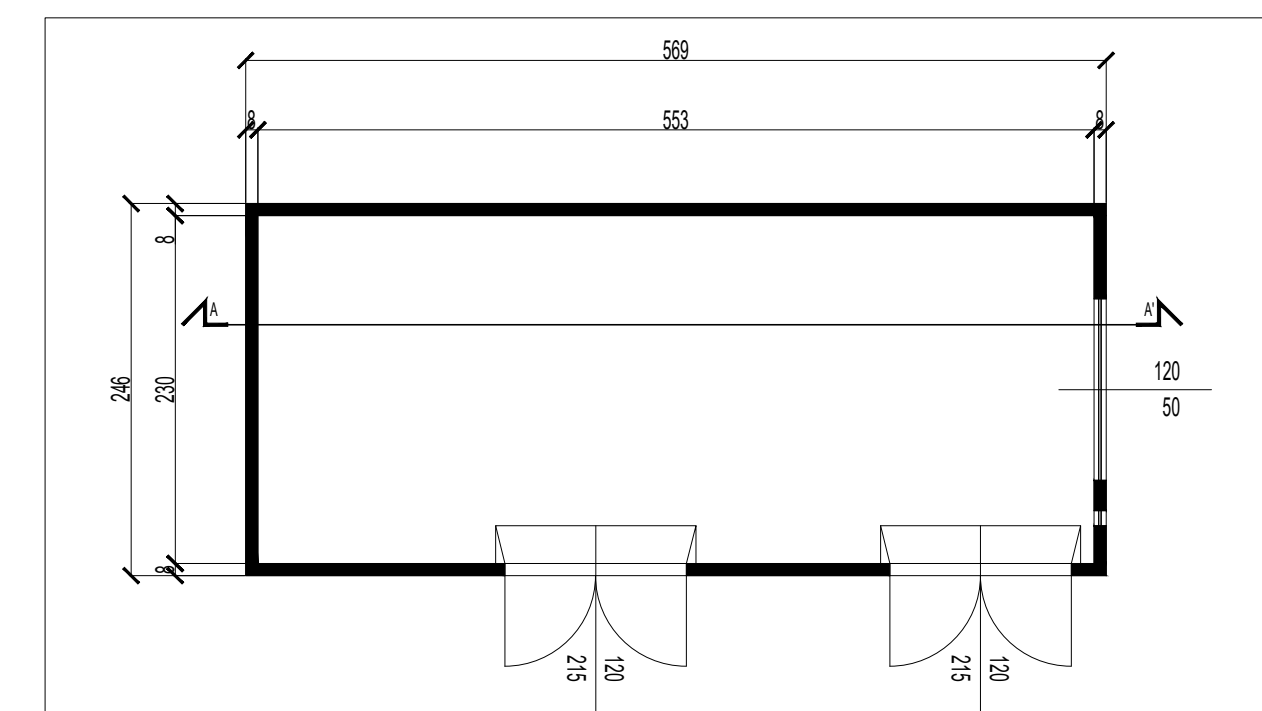
PIANTA - SCALA 1:50
