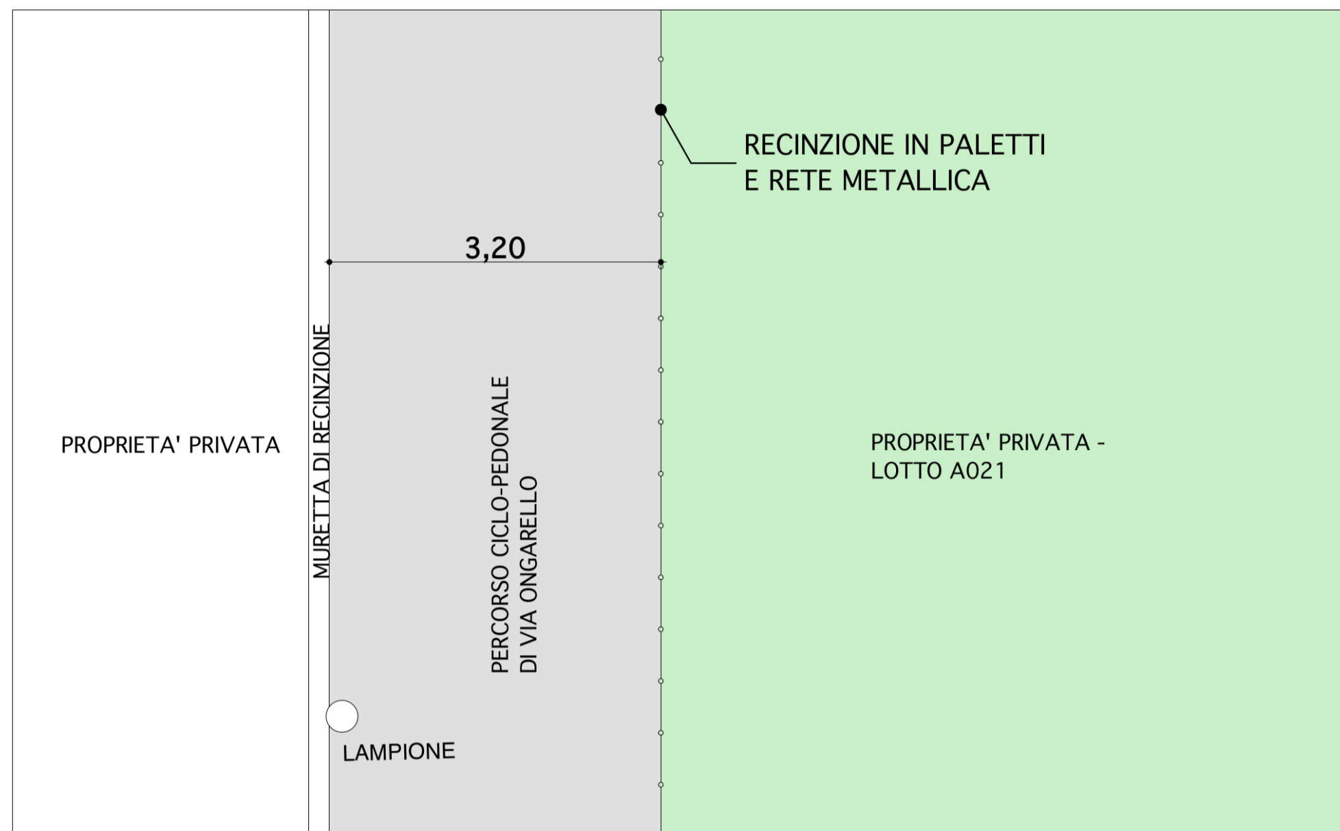
STATO DI FATTO PARTICOLARE "3" - PIANTA - SCALA 1:50
