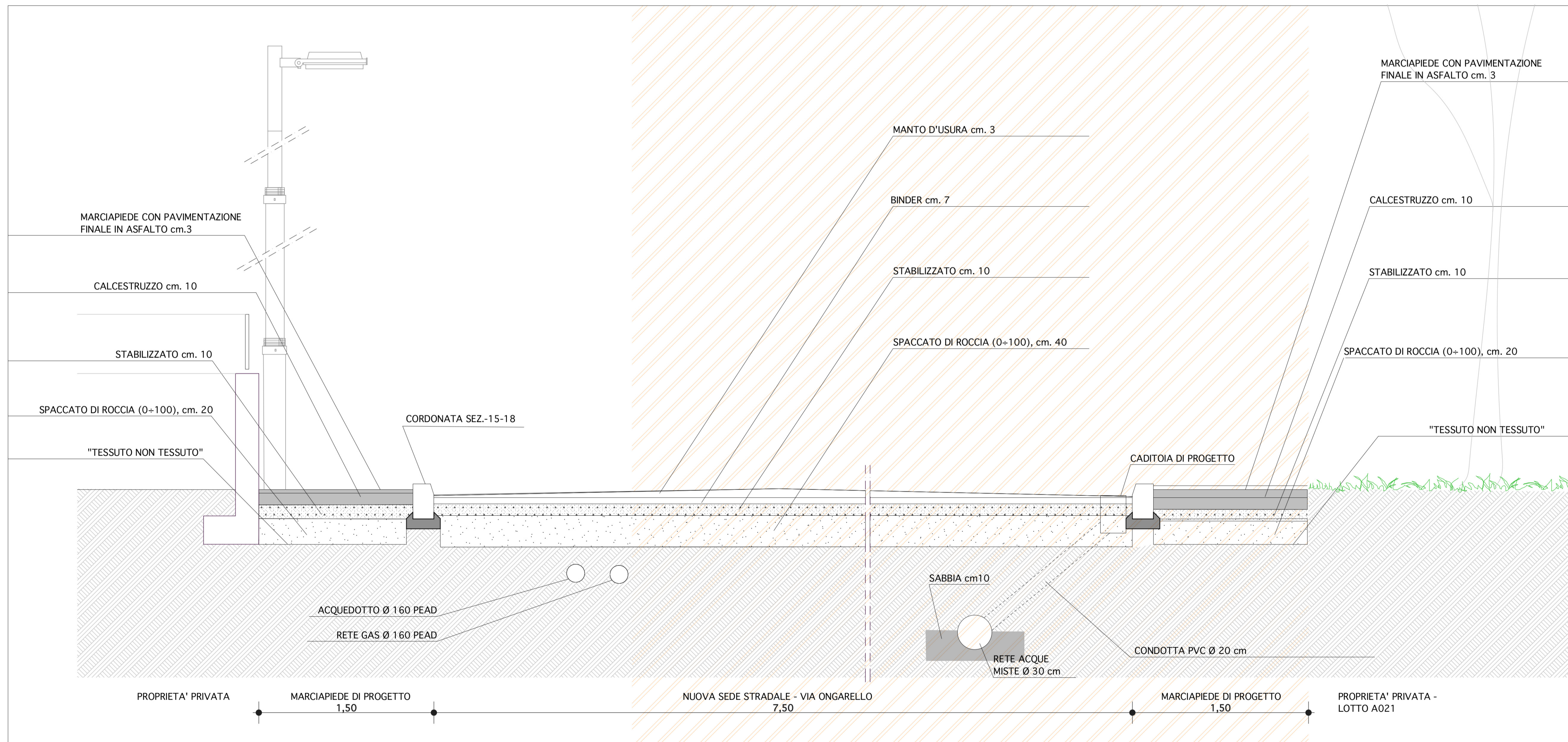
STATO FUTURO PARTICOLARE "3" - SEZIONE "C - C" - SCALA 1:20
