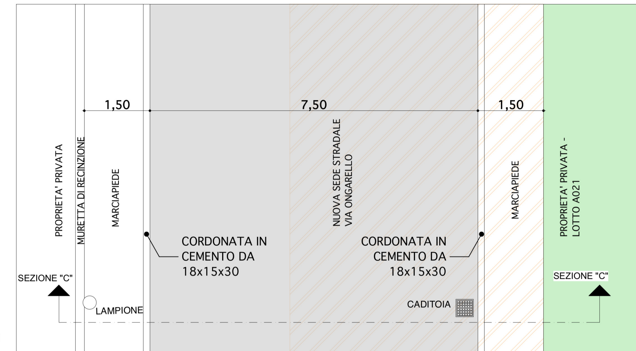
STATO FUTURO PARTICOLARE "3" - PIANTA - SCALA 1:50
