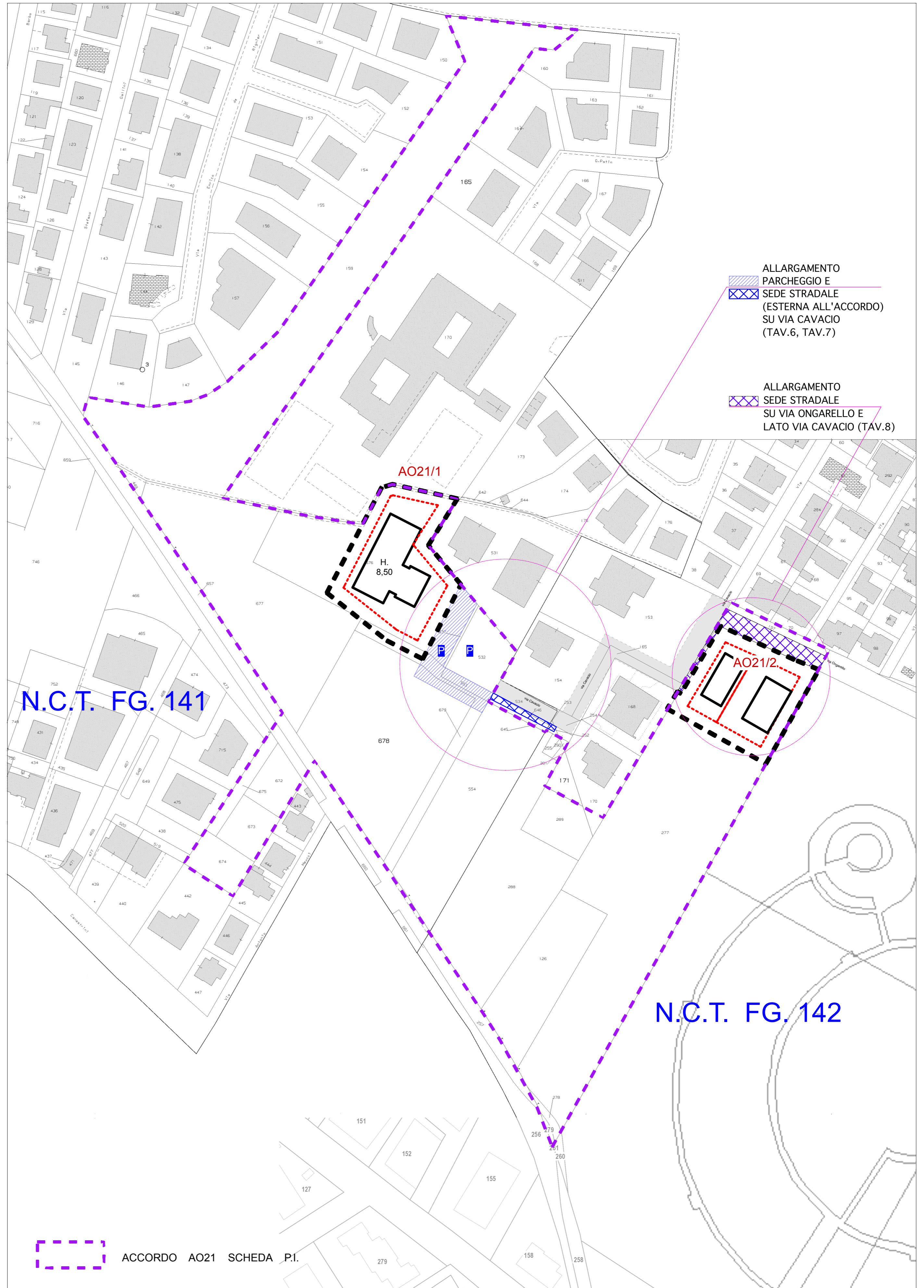
PLANIMETRIA DELLE OPERE D'URBANIZZAZIONE
