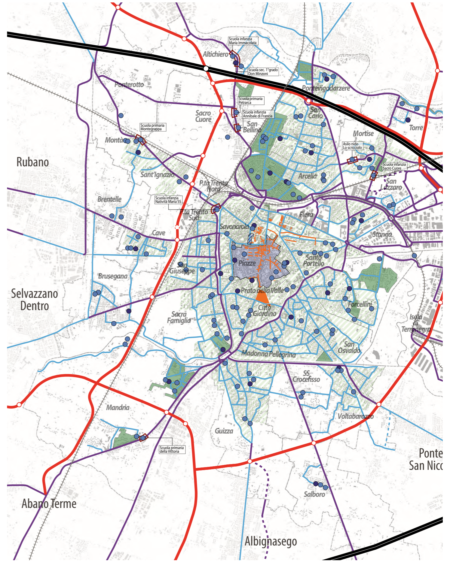
PUMS | TAVOLA DELLA REGOLAMENTAZIONE E MODERAZIONE DEL TRAFFICO: SCENARIO DI PIANO
