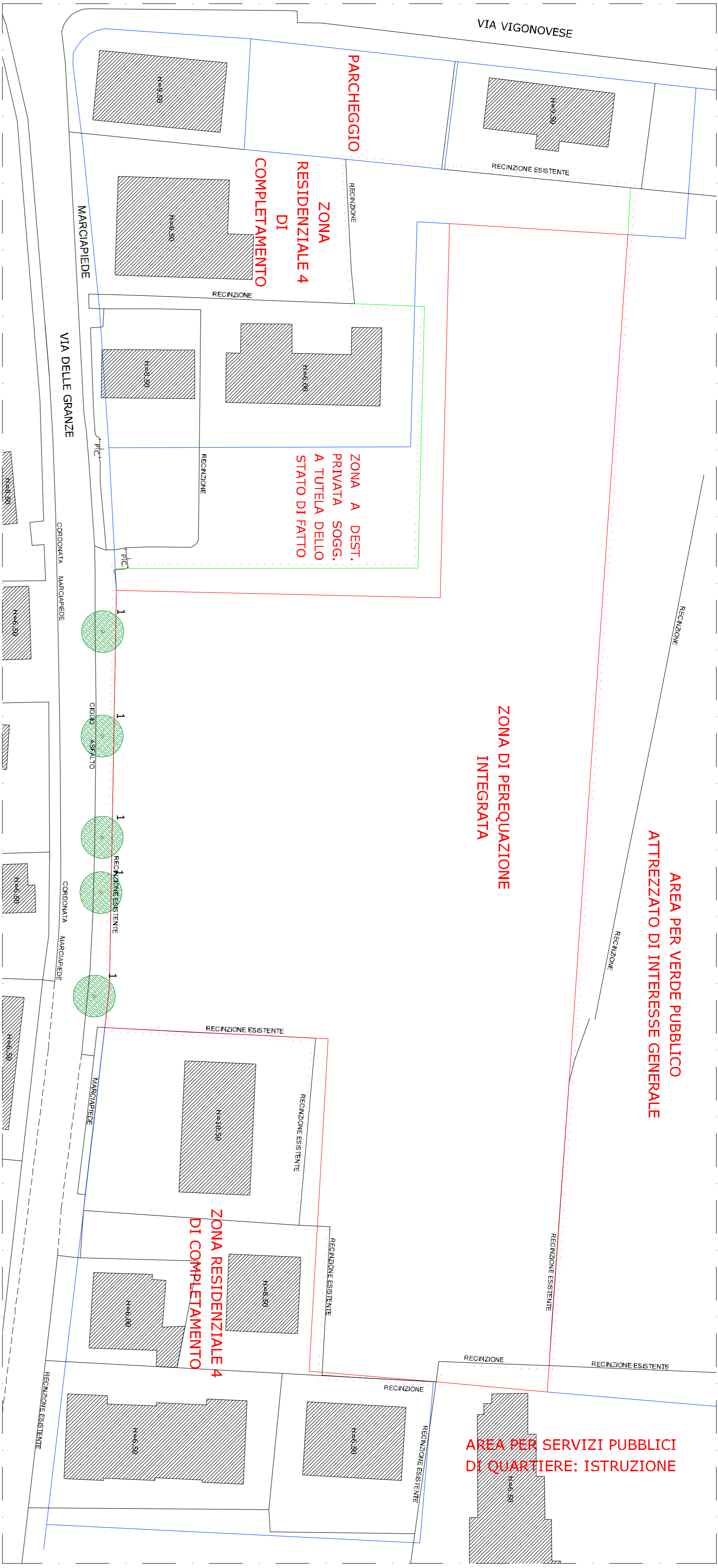
SISTEMAZIONE VERDE - STATO DI FATTO scala 1:500
