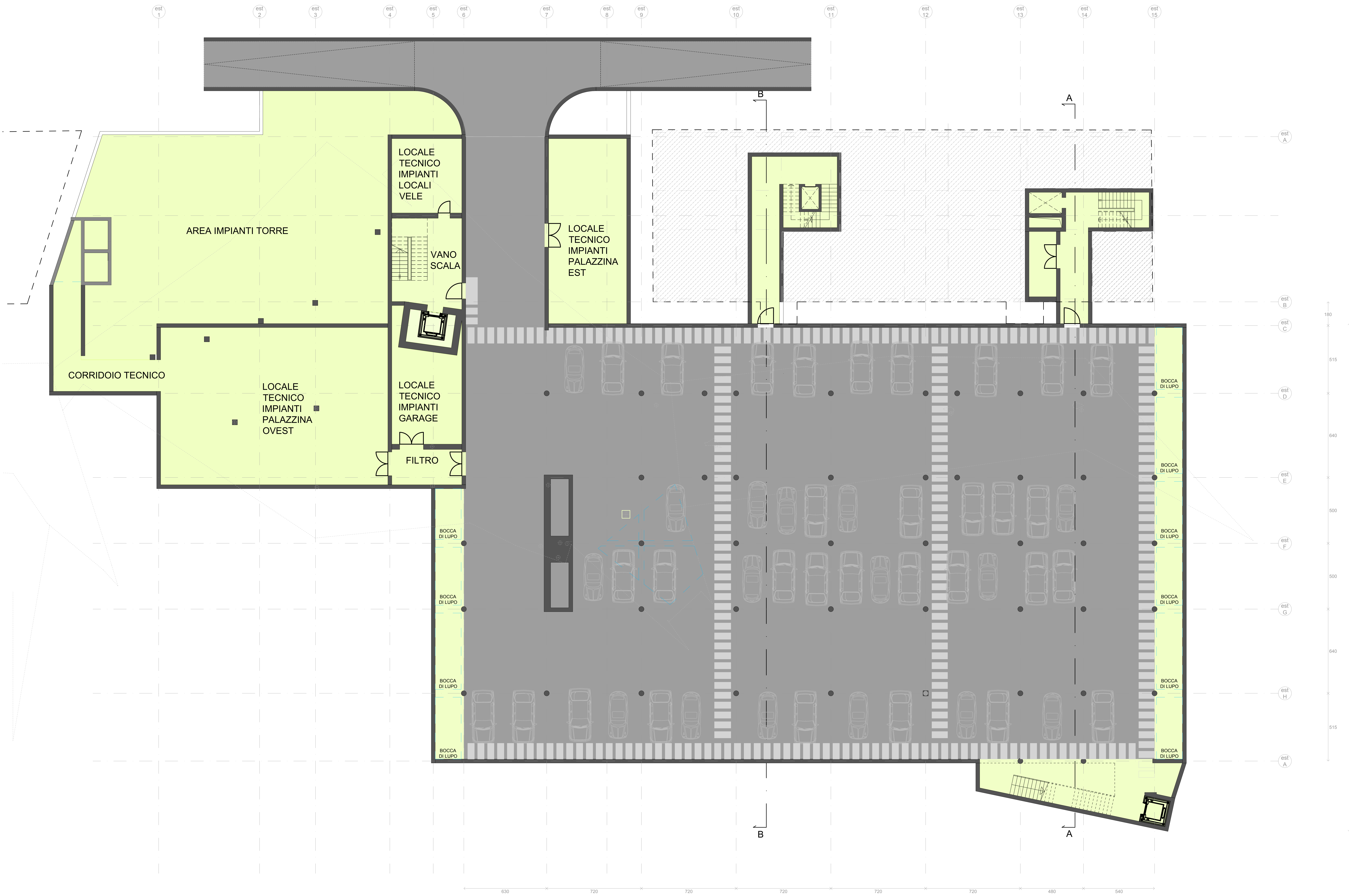
Schema Piano Interrato Palazzina Est Progetto 1:200
