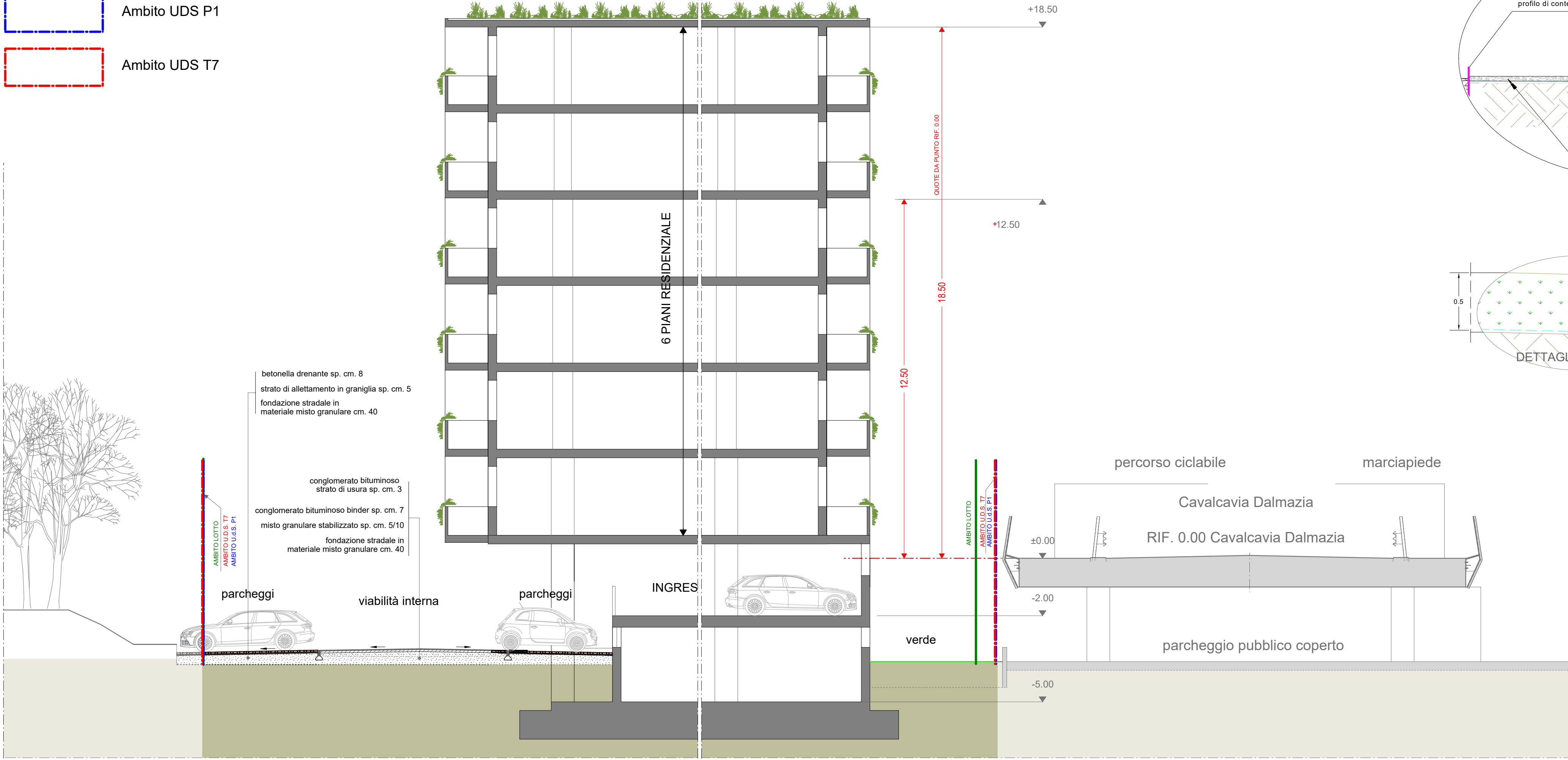
SEZIONE 3_3 DETTAGLIO PACCHETTO STRADALE E PARCHEGGI scala 1:100
