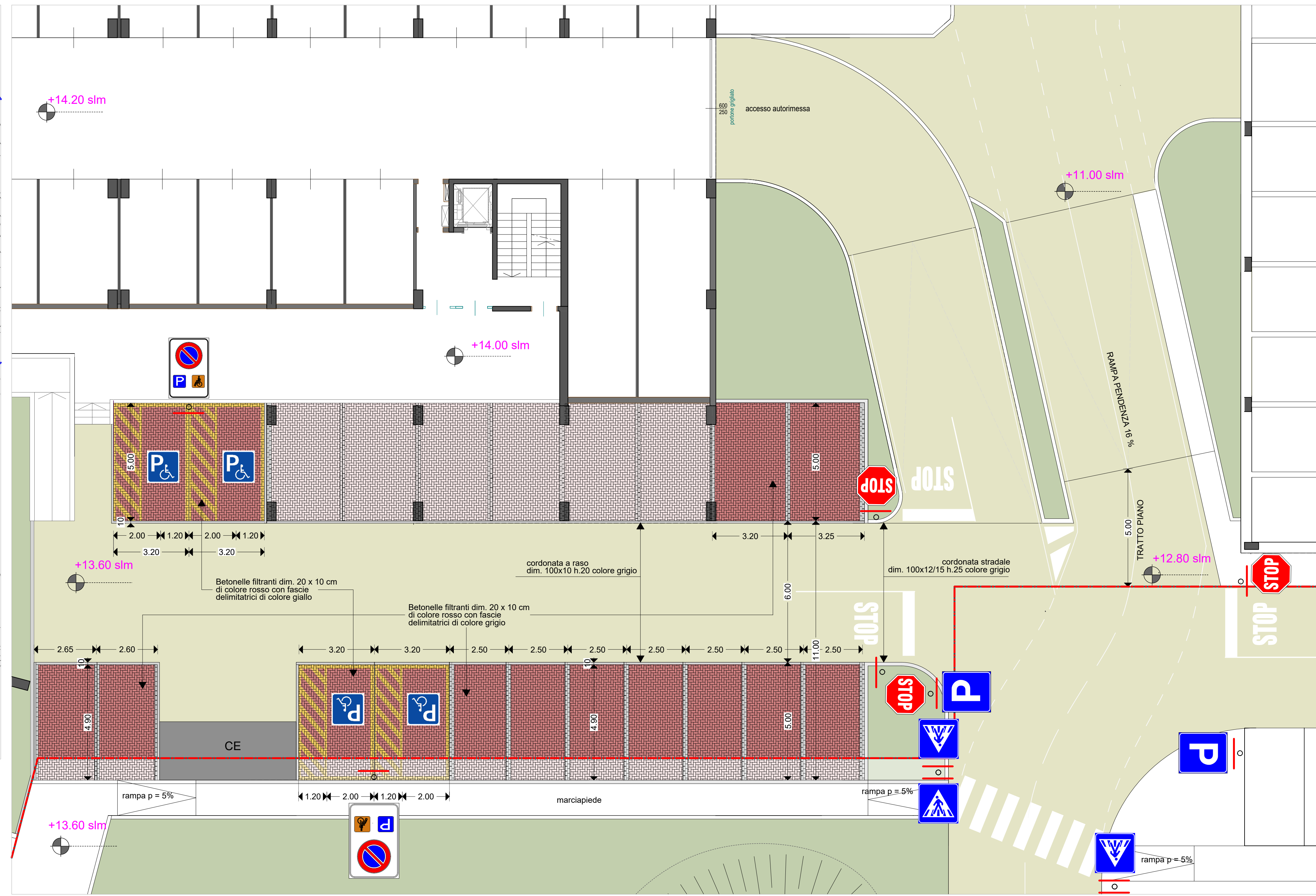
PARTICOLARE 1 SCHEMA DI POSA STALLI DI SOSTA scala 1:100
