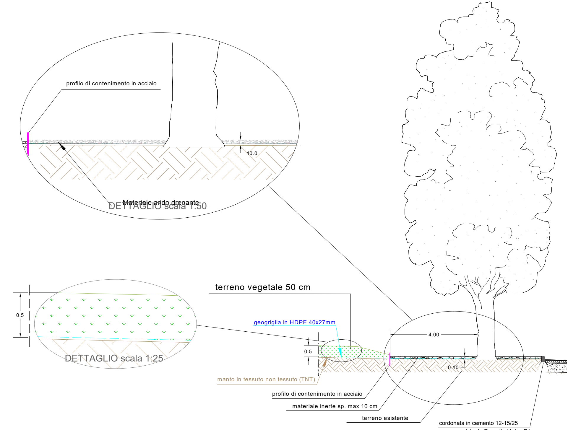
PARTICOLARE 2 REALIZZAZIONE CAPPING INTORNO ALLE ALBERATURE ESISTENTI scala 1:100
