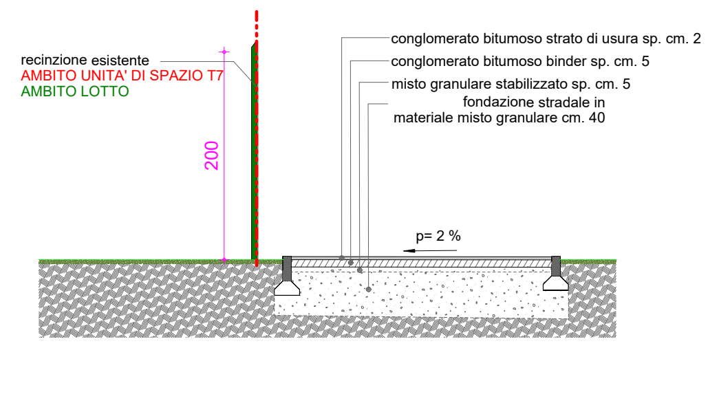
SEZIONE 2_2 DETTAGLIO PERCORSO CICLOPEDONALE scala 1:50
