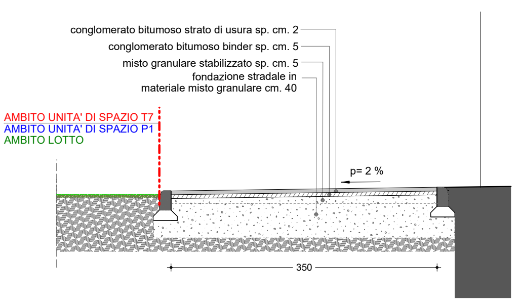
SEZIONE 1_1 DETTAGLIO PERCORSO CICLOPEDONALE scala 1:50
